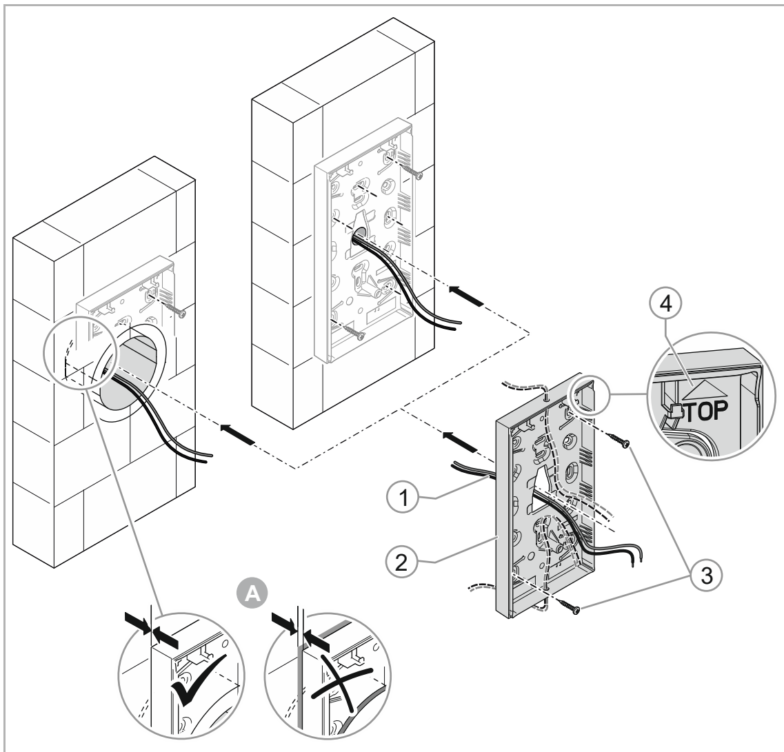
Abb. 25: Aufputzrahmen montieren
