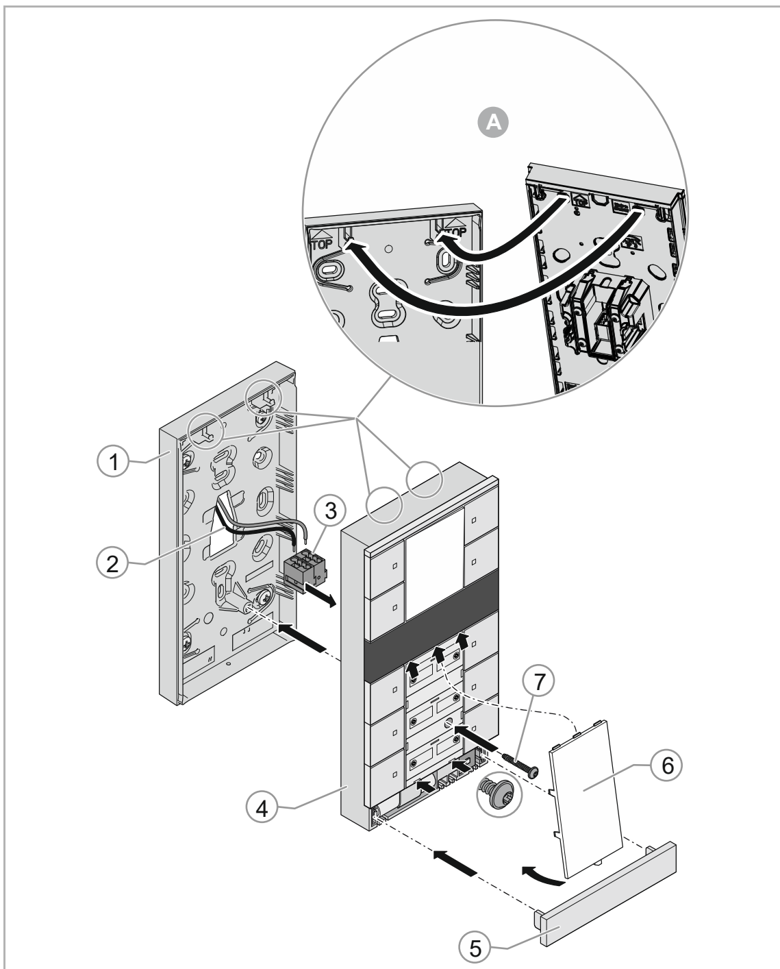
Abb. 26: Bedienelement montieren
