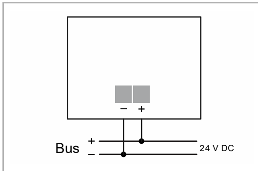
Abb. 16: Anschluss Busankoppler
