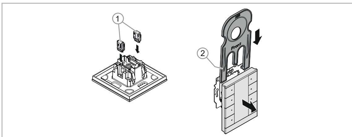
Abb. 5: Entnahmeschutz
