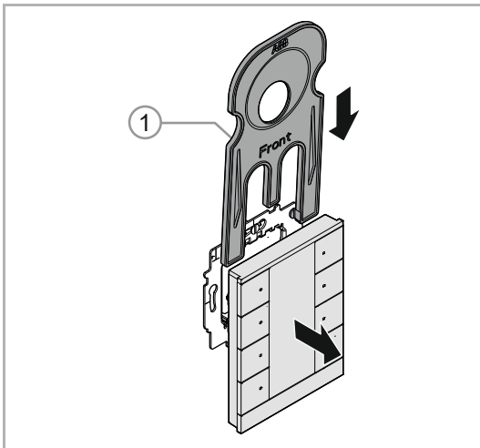
Abb. 22: Demontage Entnahmewerkzeug
