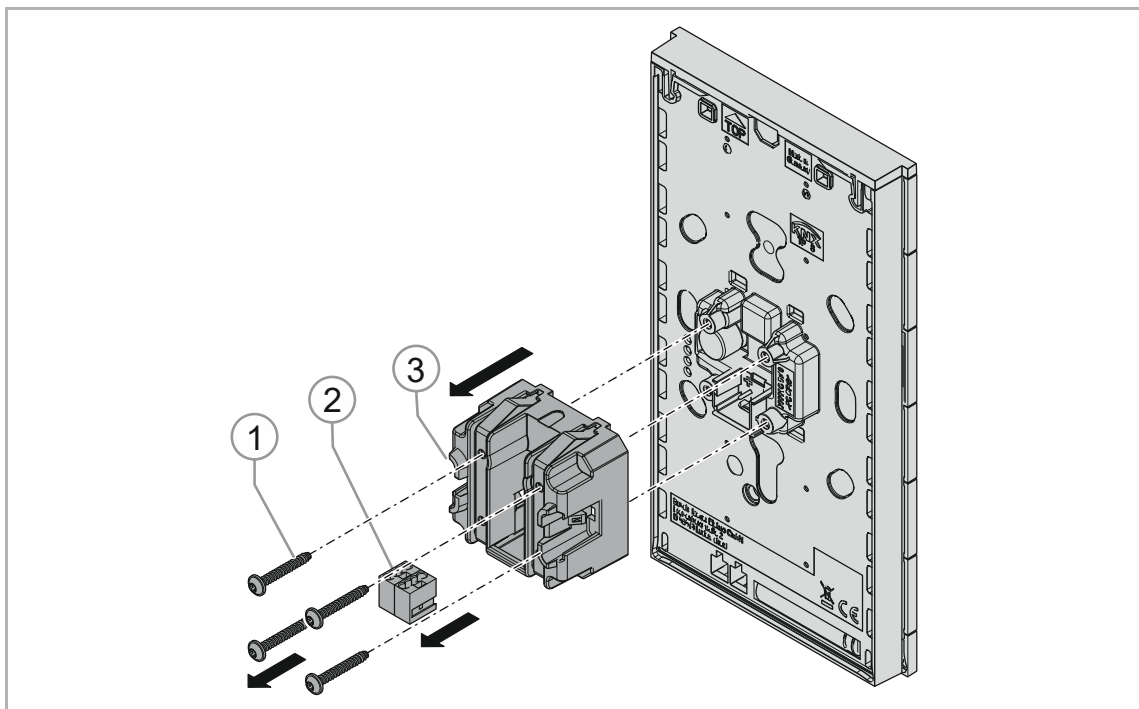
Abb. 23: Bedienteil vorbereiten
