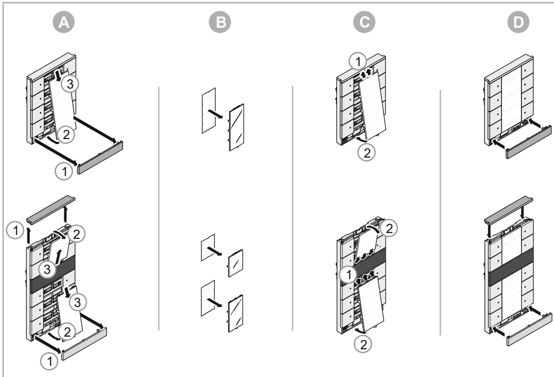
Abb. 27: Beschriftungs-Einleger
