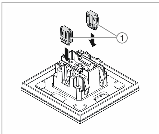
Abb. 17: Montage Entnahmeschutz
