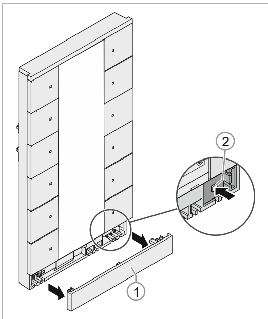
Abb. 21: Programmierleiste
