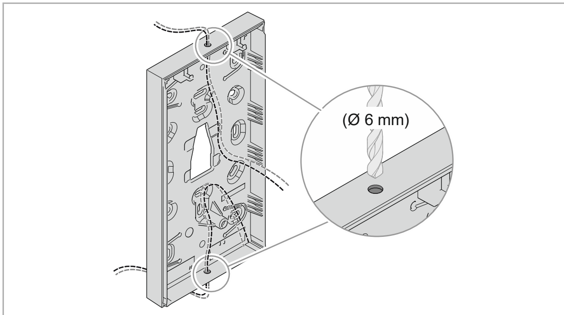
Abb. 24: Alternative Buskabelführung
