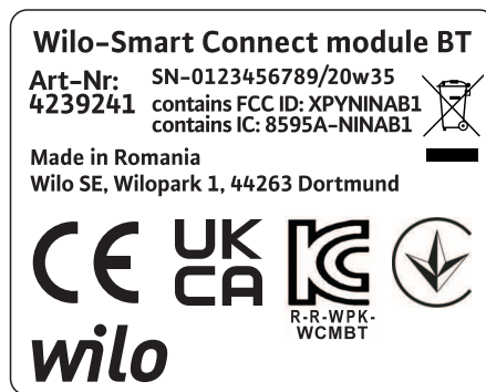
Fig. 1: Príklad typového štítku – statický PIN
