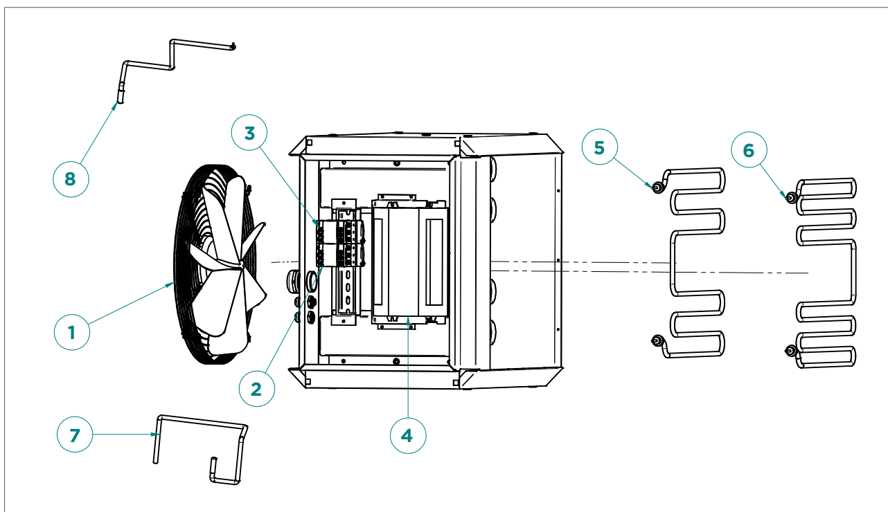
Figure 16 - Vue éclatée de EH
