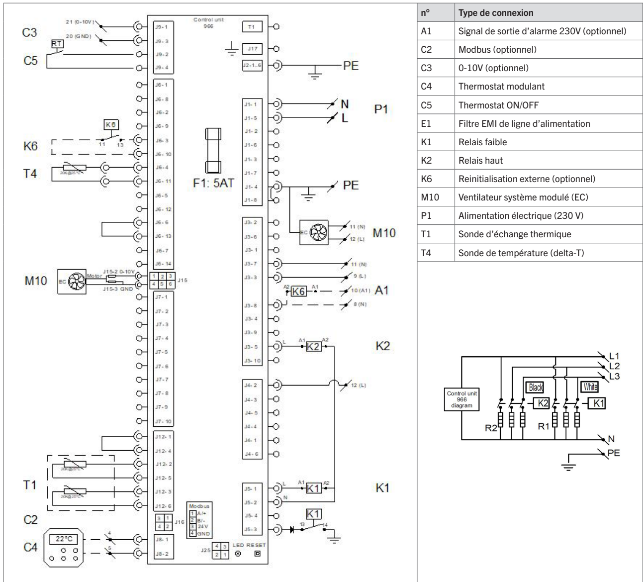
Figure 14 - Schéma de câblage EH-EC
