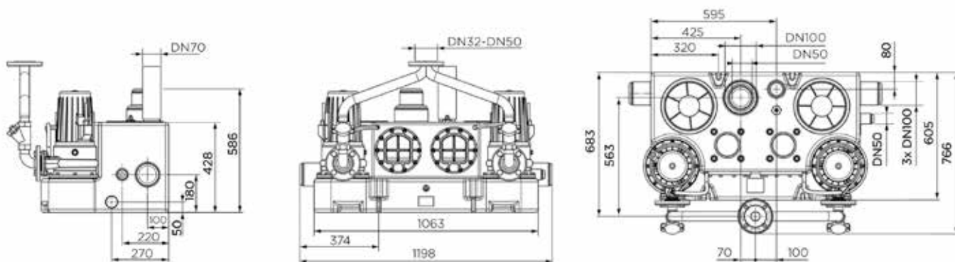
Afmetingen (mm)
