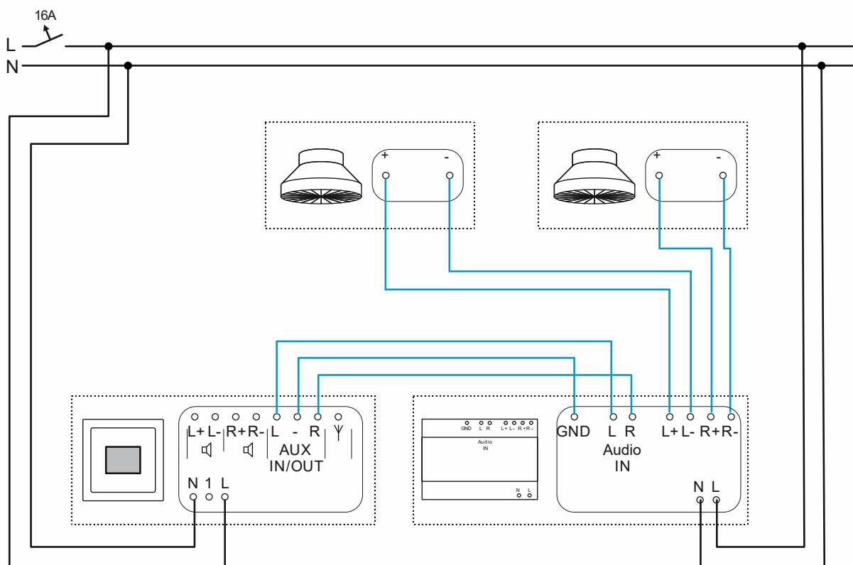
Рис. 77: Радио с усилителем мощности и 2 громкоговорителями: подключение
