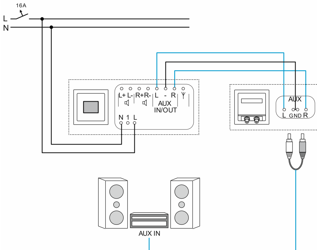
Рис. 78: Радио и HiFi-систем: обзорная схема
