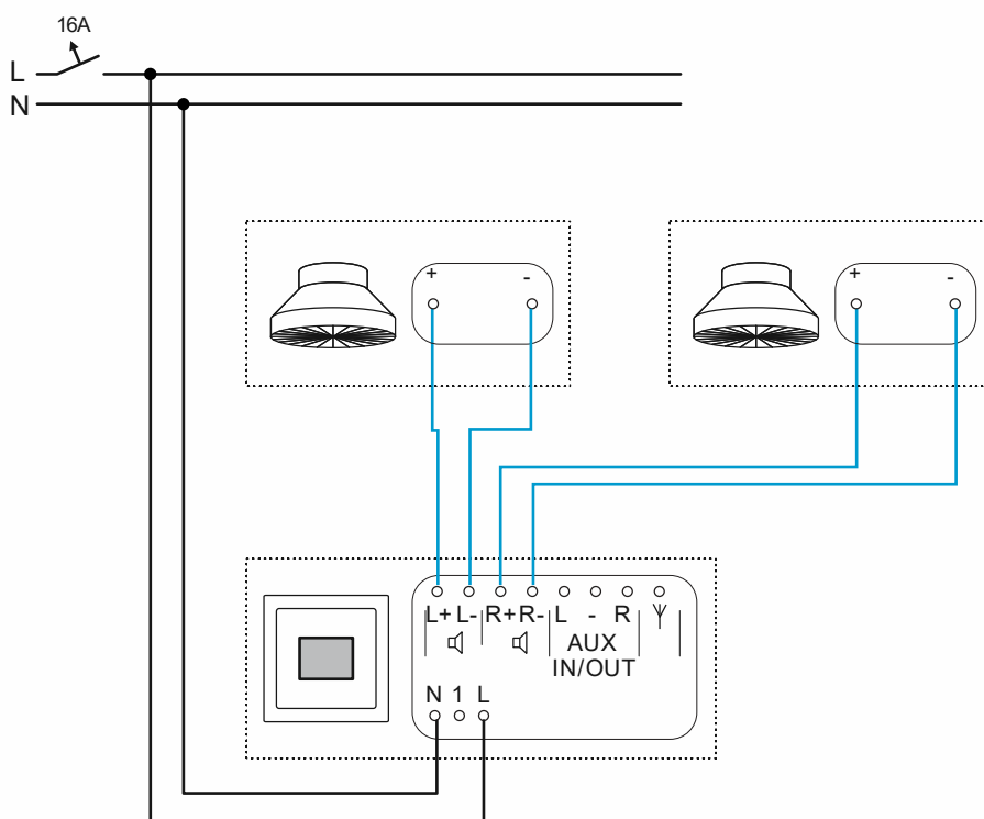
Рис. 75: Радио с 2 громкоговорителями: подключение
