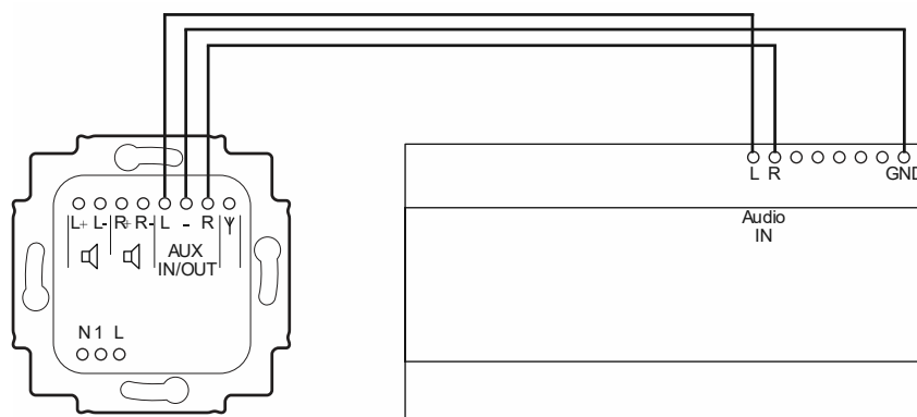
Рис. 11: Подключение внешнего усилителя мощности
