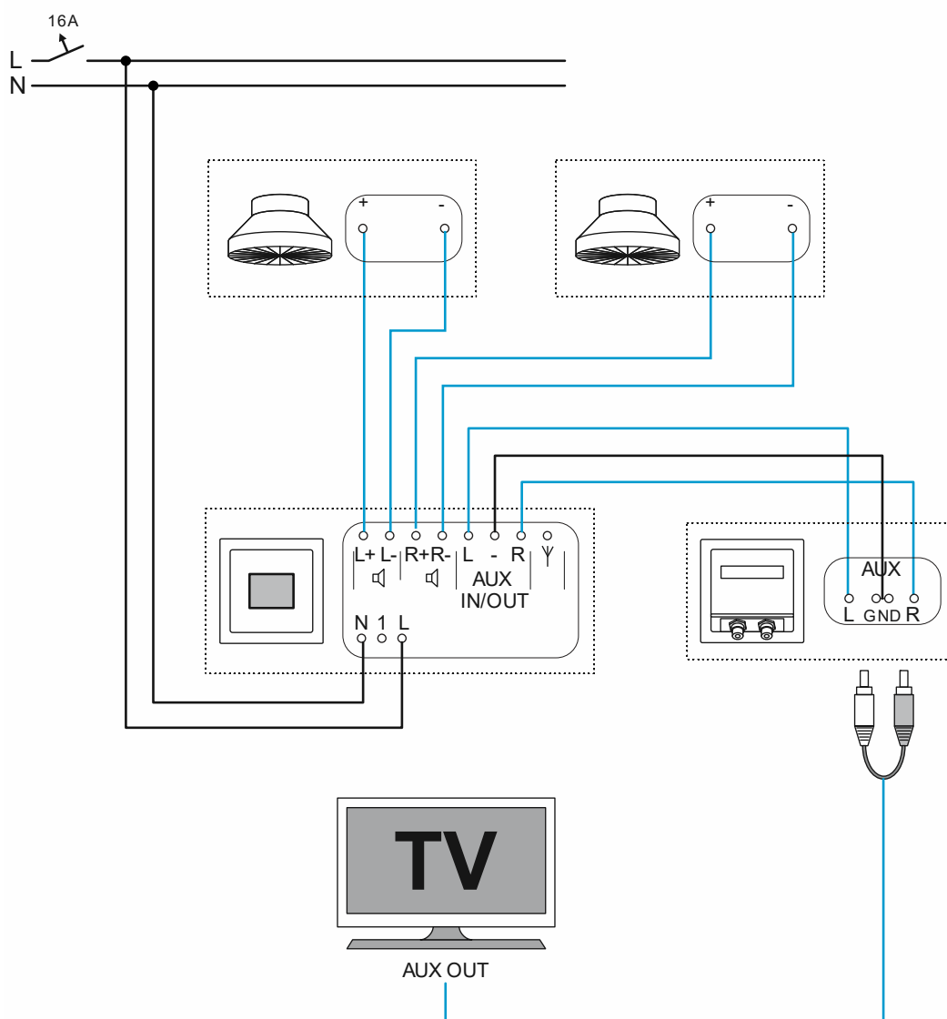
Рис. 81: Радио и ТВ: подключение
