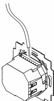
Рис. 3: Подключение кабелей громкоговорителя/сигнальных проводов
