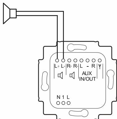
Рис. 9: Подключение громкоговорителя для работы в моно-режиме
