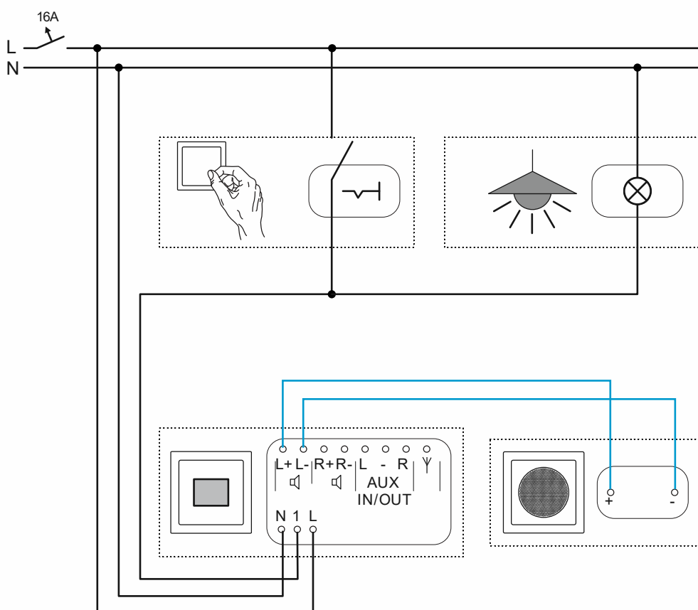
Рис. 70: Монтажный комплект и управления с вспомогательного устройства: подключение
