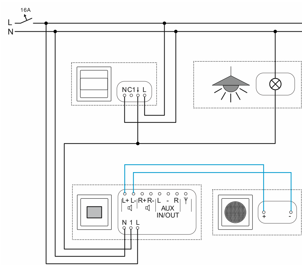
Рис. 72: Монтажный комплект и датчик движения: подключение
