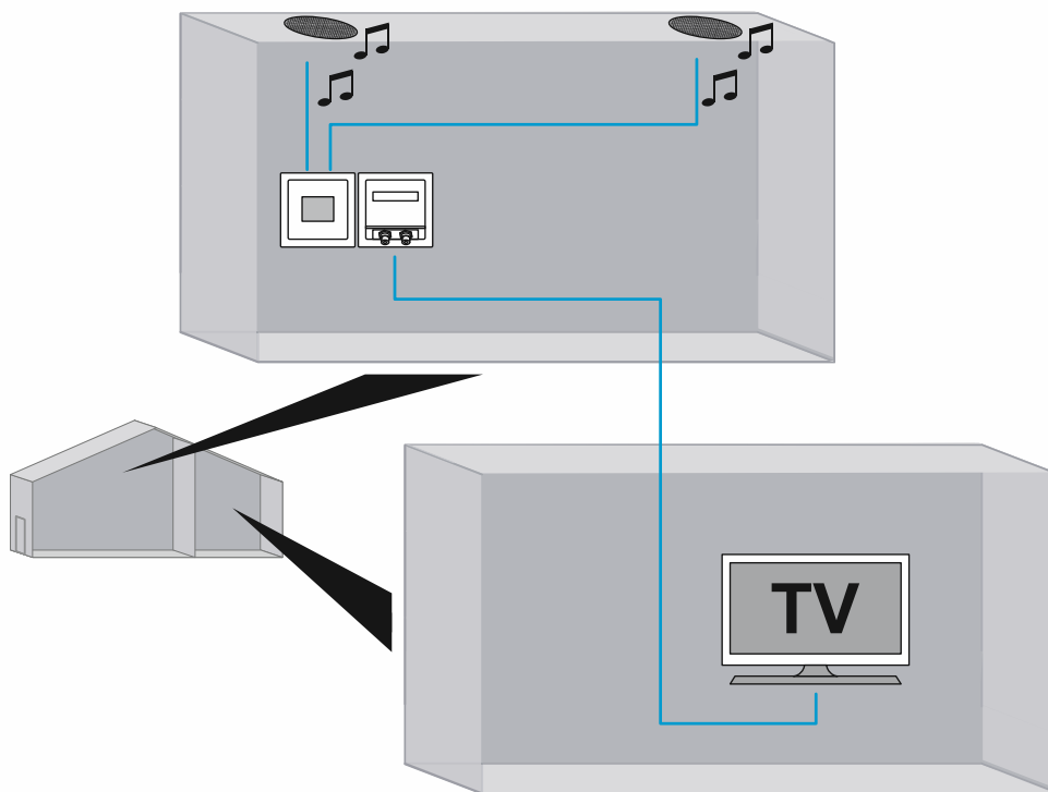
Fig. 80 : Radio encastrée avec TV : présentation
