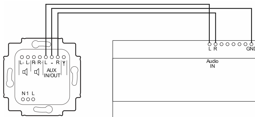
Fig. 11: Connecteur AUX d'un amplificateur de puissance
