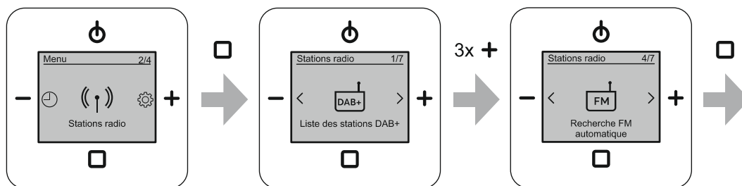
Fig. 41 : Recherche automatique de stations FM
