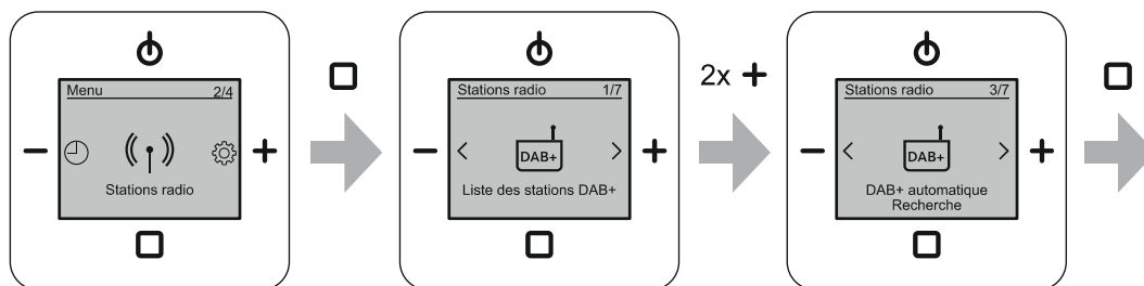
Fig. 40 : Recherche automatique de stations DAB+
