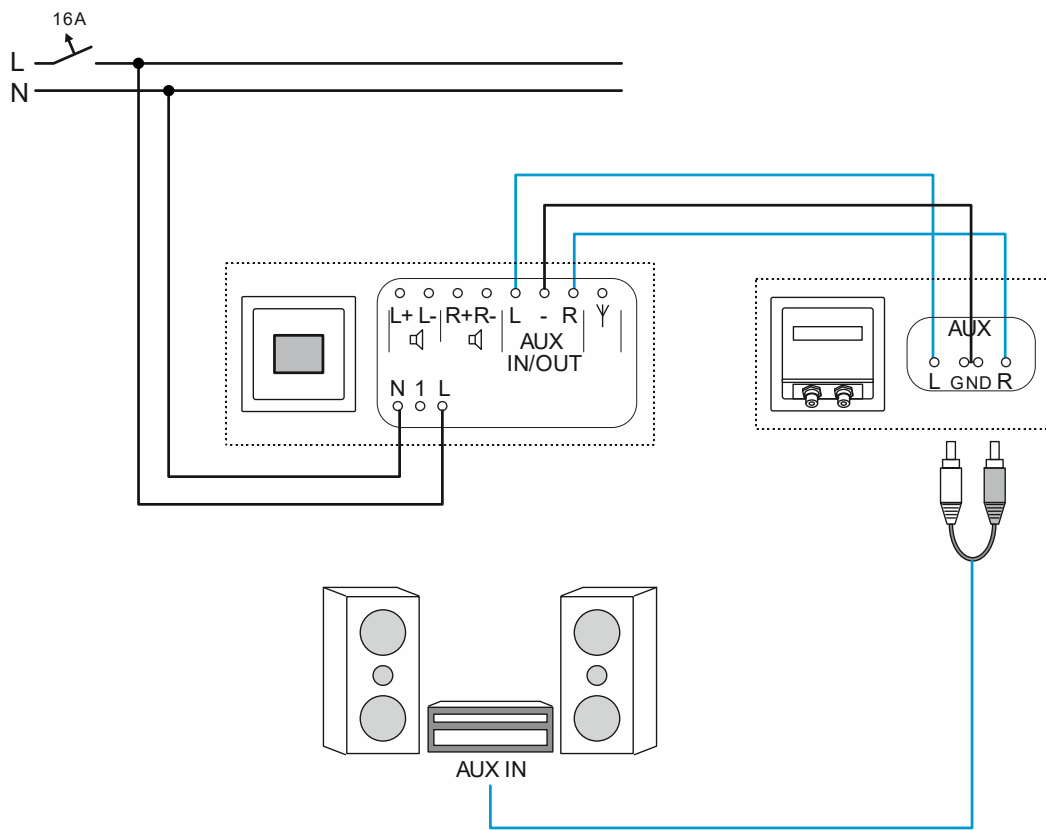
Fig. 79 : Radio encastrée avec chaîne Hi-Fi : raccordement
