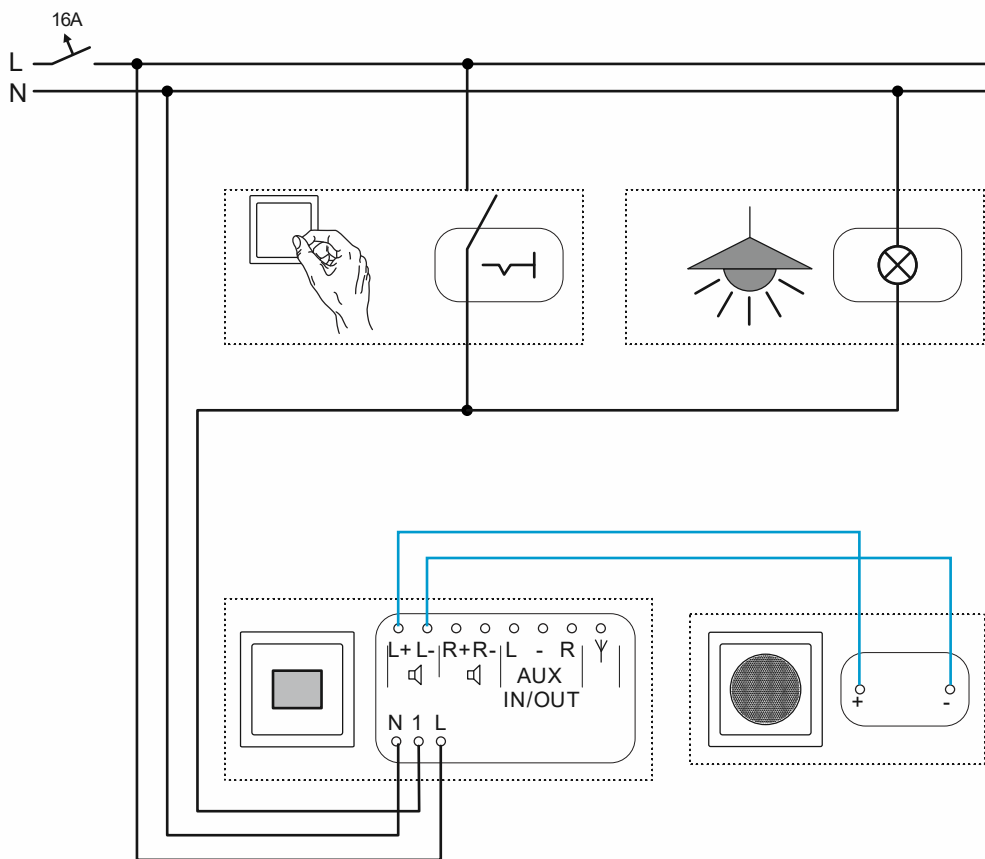
Fig. 70 : Kit de montage avec commande par poste auxiliaire : raccordement
