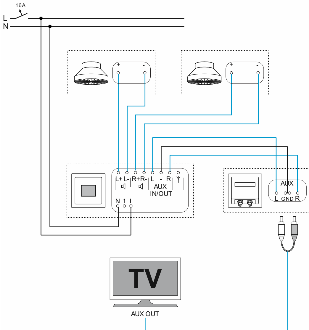
Fig. 81 : Radio encastrée avec TV : raccordement
