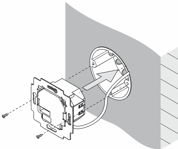
Fig. 5 : Montage du mécanisme encastré
