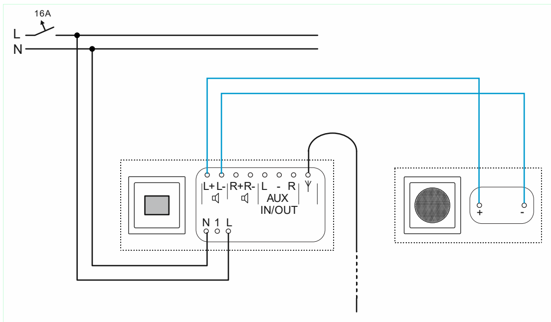
Fig. 68 : Raccordement du kit de montage (antenne flexible, 90 cm de long environ)
