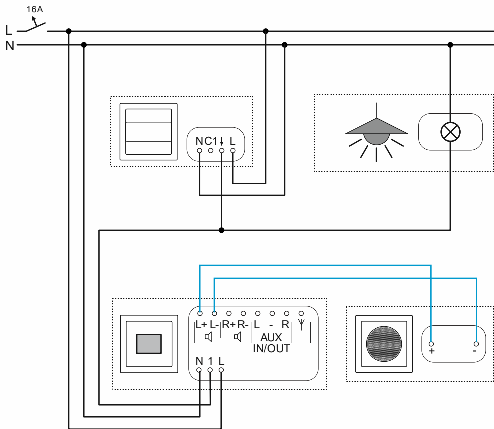
Fig. 72 : Kit de montage et détecteur de mouvement : raccordement
