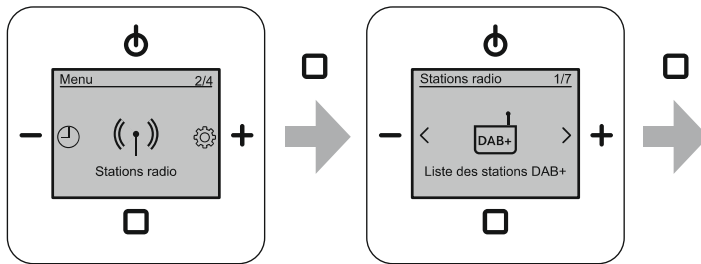
Fig. 38 : Afficher la liste des stations DAB+
