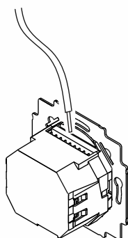
Fig. 3 : Raccordement des câbles haut-parleurs / lignes de signaux
