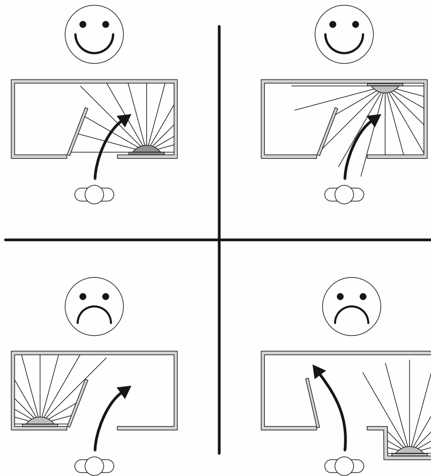
Fig. 73 : Exemples de positionnement favorable et défavorable du détecteur de mouvement (positionnement avec la radio)
