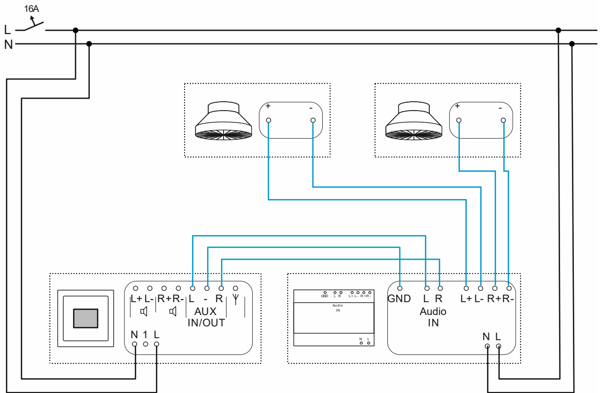
Fig. 77 : Radio encastrée avec amplificateur de puissance et 2 haut-parleurs au plafond : raccordement
