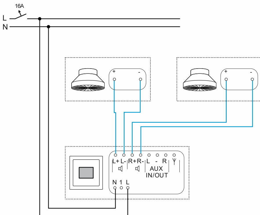
Fig. 75 : Radio encastrée avec 2 haut-parleurs au plafond : raccordement
