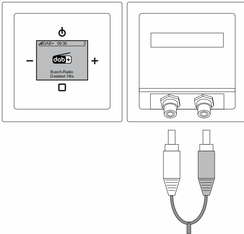
Fig. 12 : Extension AUX Cinch
