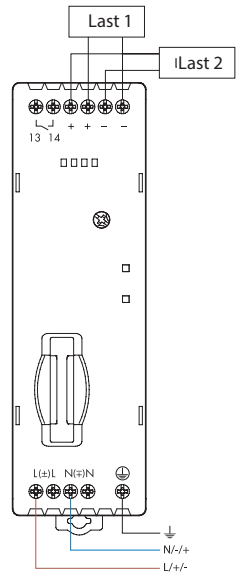
78.1D - Aansluitschema
