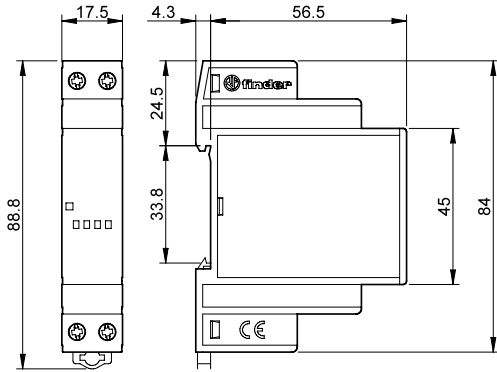
Type 78.36 / 78.50 / 78.60 Schroefaansluiting
