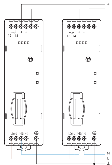
Serieschakeling voor spanningsverdubbeling
