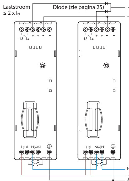
Parallelschakeling voor grotere stroom
