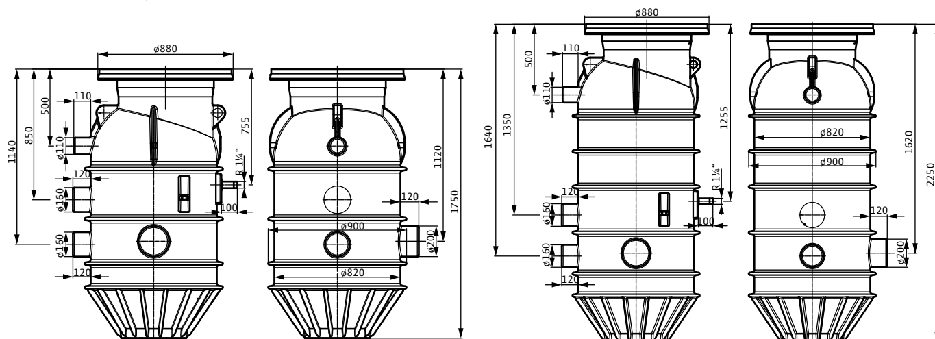
Sl. 2.: Crtež sa dimenzijama
