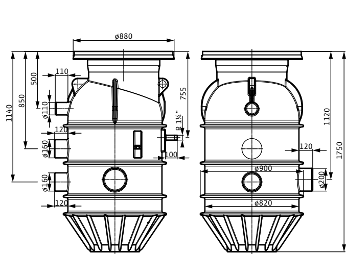
Sl. 2: Merska risba
