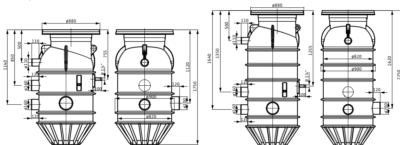
Slika 2.: Mjerni crtež
