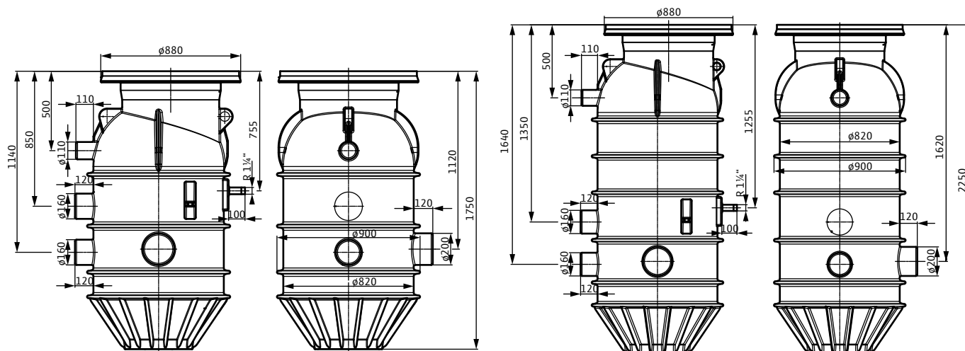
Bild 2.: Måttskiss
