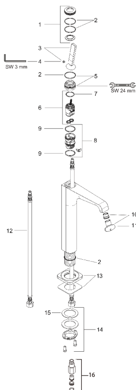
部品リスト
