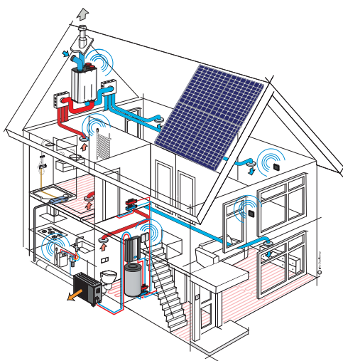
Plaatsing HP-S in woningbouw
