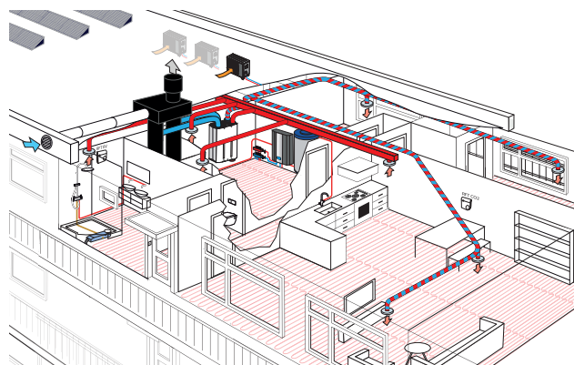
Plaatsing HP-S in een appartements gebouw
