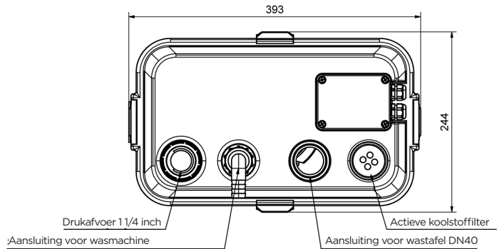
Afmetingen (mm)
