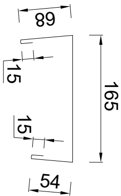
Gootbladvanger Doorsnede. Schaal 1:5
