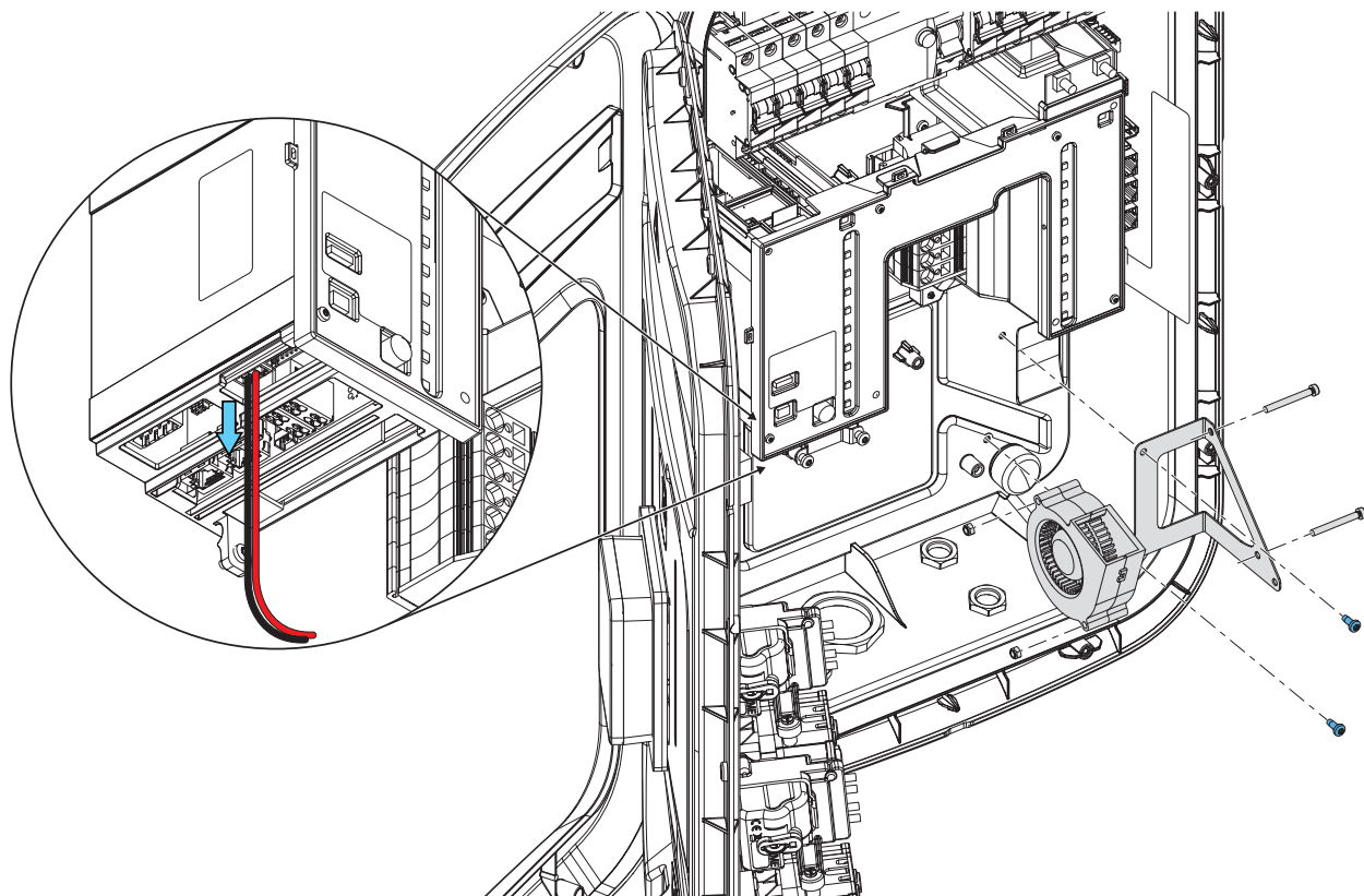
Figure 79. Fan overview
