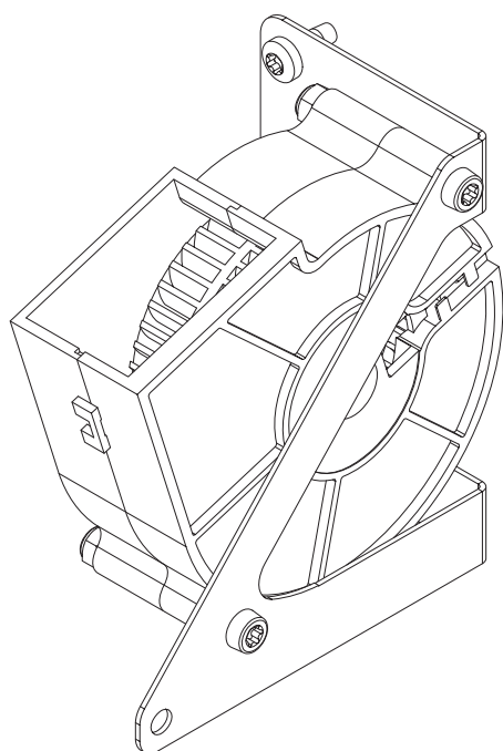
Figure 79. Fan overview
