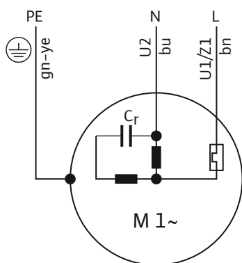
Fig. 7: Aansluitschema 1~motor
