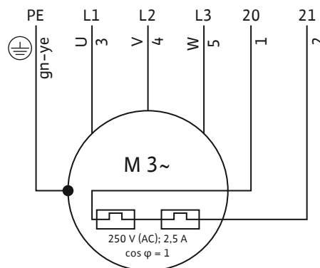
Fig. 8: Aansluitschema 3~motor
