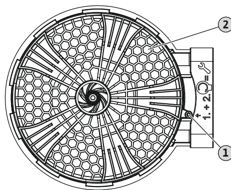
Fig. 9: Grondplaat demonteren
