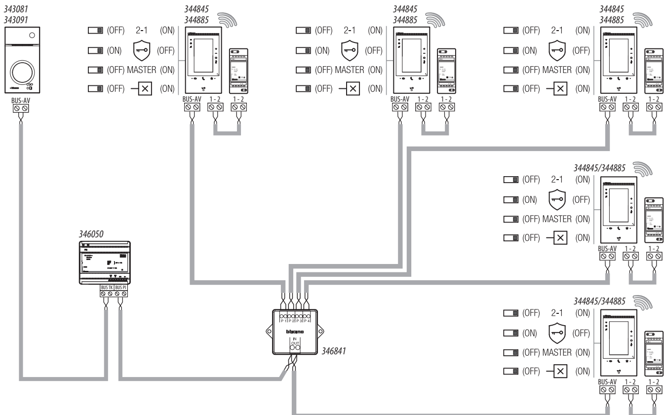
SCHEMA 7 - VOORBEELD VAN EEN EENGZINS INSTALLATIE MET 5 CLASSE 300EOS WITH NETATMO
