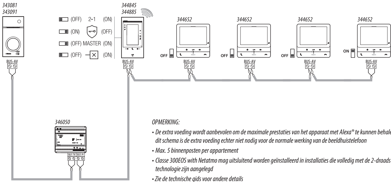
SCHEMA 6 - VOORBEELD VAN EEN EENGZINS INSTALLATIE
