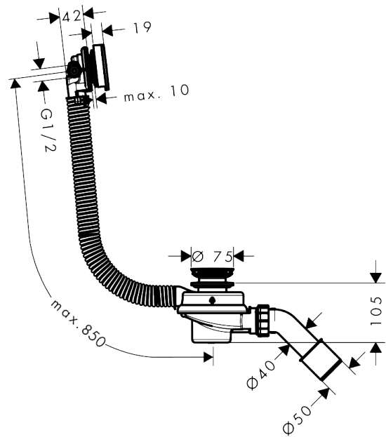
Maattekening
