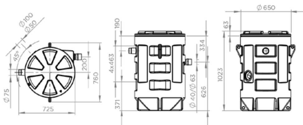
Afmetingen (mm)
