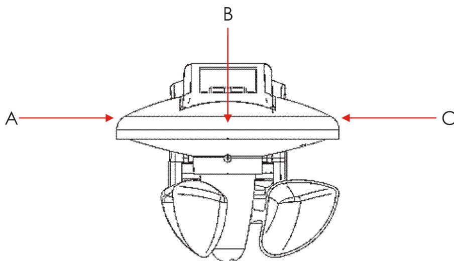
Abbildung 1: Helligkeitssensoren.
