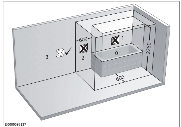
Elektrische veiligheidszones in de badkamer
