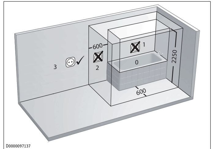
Zones de protection électrique dans la salle de bains
