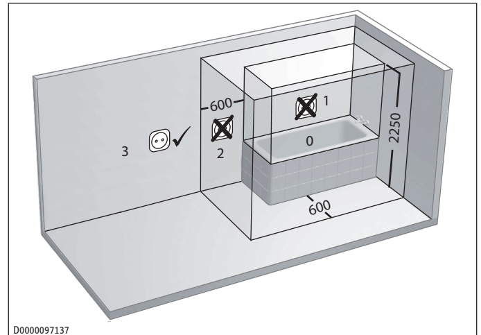
Elektrische Schutzbereiche im Badezimmer
