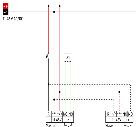
Schakelschema
