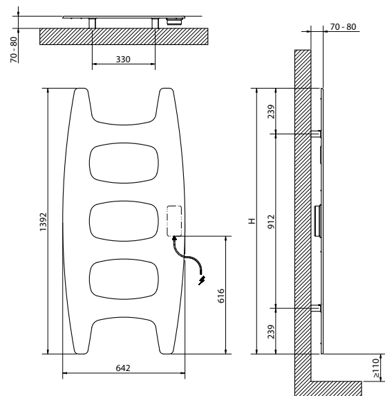
Detail control unit en positie snoer
