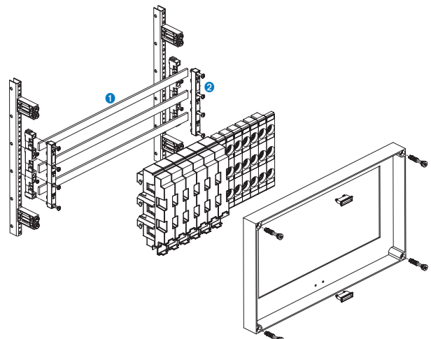
Abb. 3: D-Reiter-Sicherungssockel, 3-polig, montiert auf Sammelschienen-Träger. Phasenmittenabstand 60 mm, mit Cu-Sammelschienen-System 20x5 oder 30x10 mm
