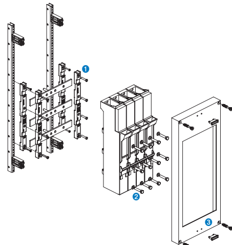
Abb. 2: Normfeld-Einbausätze mit NH-Sicherungstrennleisten, 3-polig, vertikal montiert auf Sammelschienen-Träger. Phasenmittenabstand 100 mm, mit Cu-Sammelschienen-System 30x5 oder 30x10 mm
