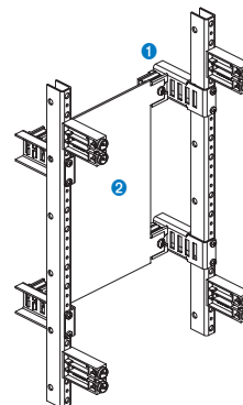
Abb. 8: Montageplatte mit Absenkbügelset 1) Absenkbügelset 2) Montageplatte
