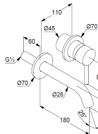
Maßzeichnung/ Dimensional drawing
