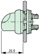
Selector M22-W.K...
