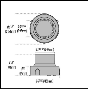
3109879 Inbouwdoos CRICKET+ 10
