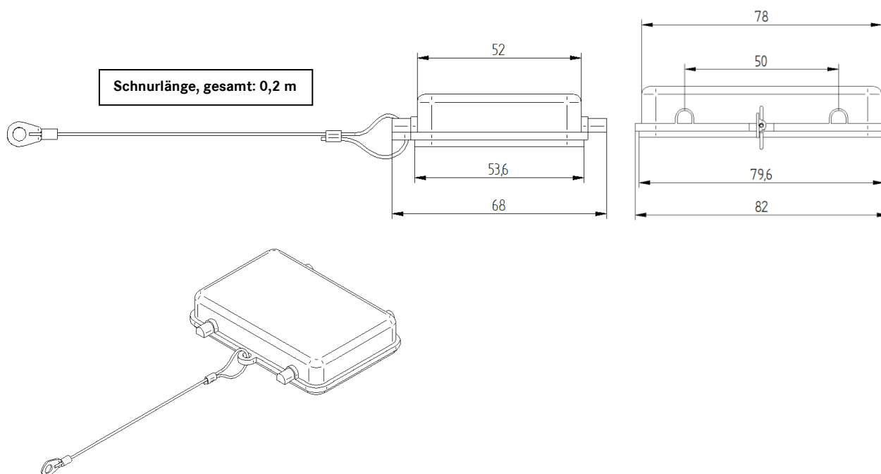
EPIC® H-A 32 KDBF (mit Fangschnur), 10481500
