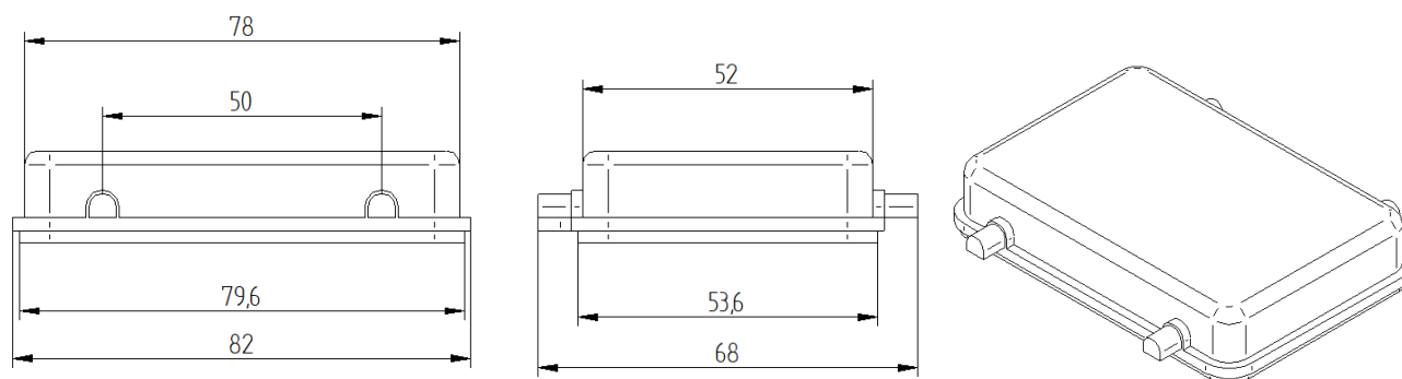
EPIC® H-A 32 KDB (ohne Fangschnur), 10481700
