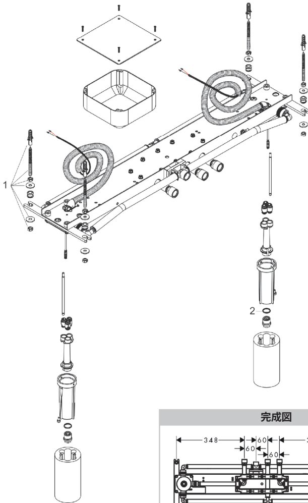
製品分解図
