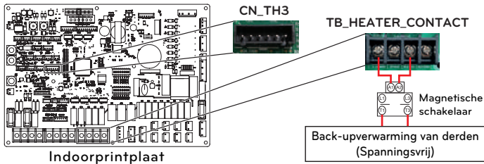
Indoorprintplaat
