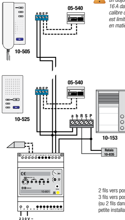
fig.1: schéma de raccordement complet
