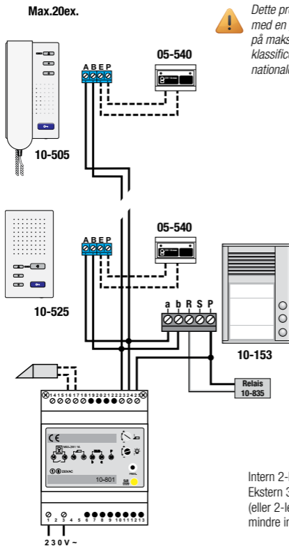
fig.1: komplet tilslutningsskema
