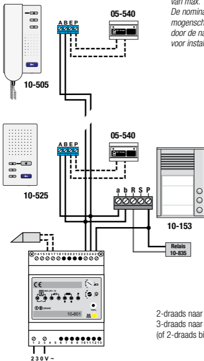
fig.1: compleet aansluitschema
