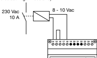
Fig.3: tilslutning af et lyskredsløb (230V ~) til STRØMFORSYNING 20
