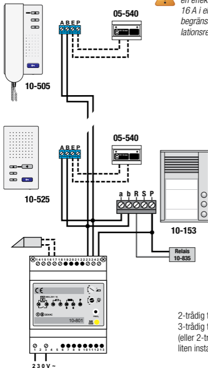
fig.1: komplett kopplingschema
