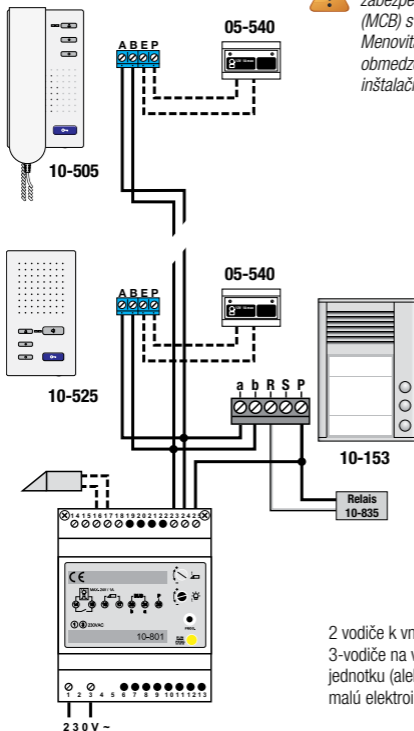
Obr. 1 Úplná schéma zapojenia
