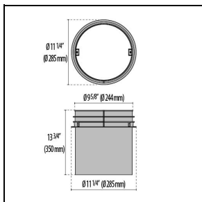
3111135 Inbouwdoos
