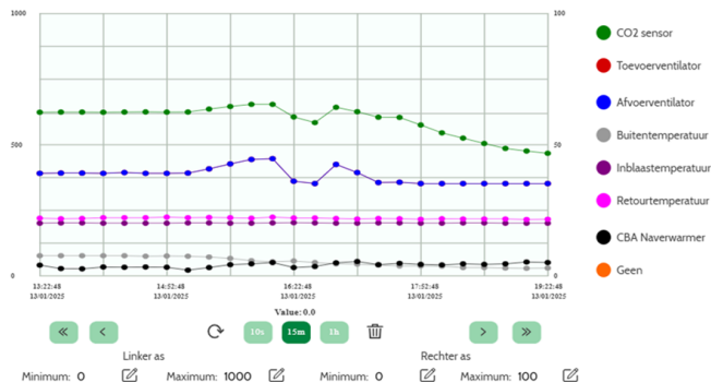
Signaalanalysator (trend)
