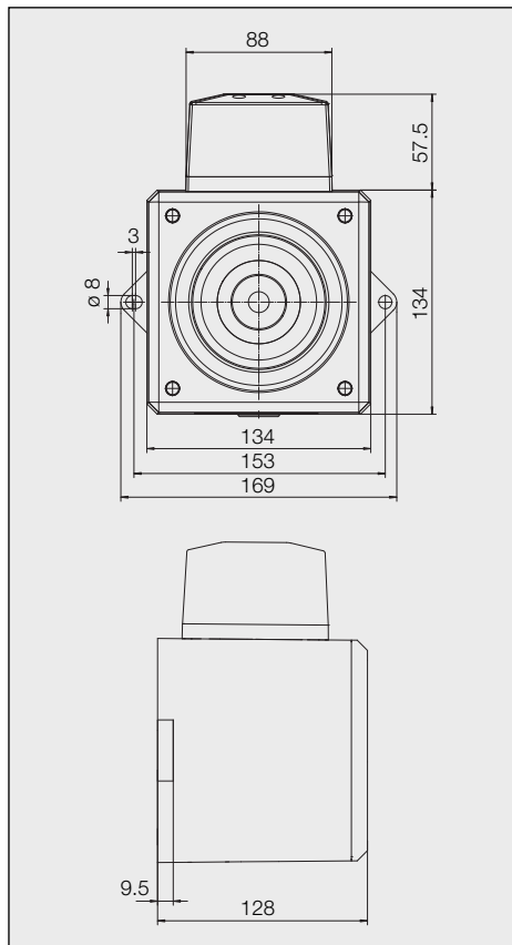
Dimensions AXL05
