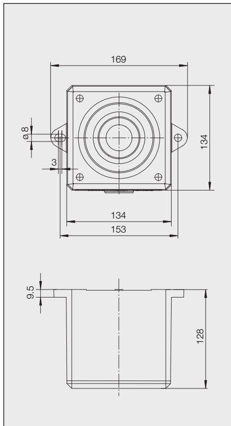
Dimensions AX05
