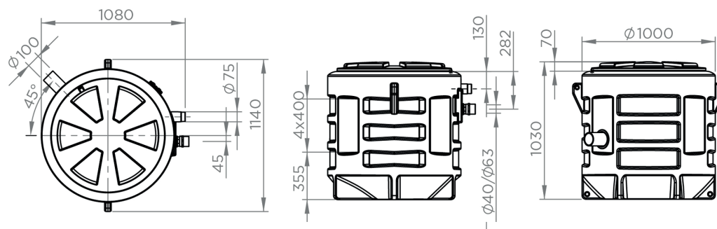
Afmetingen (mm)
