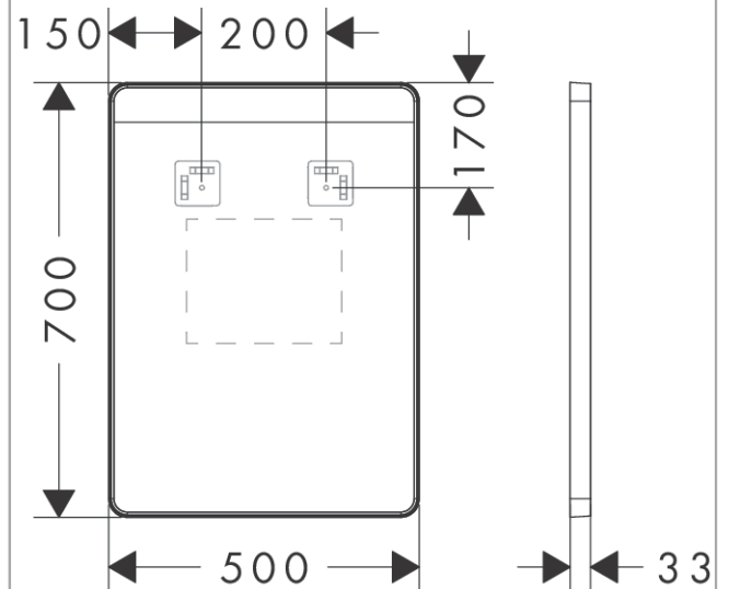
Maattekening
