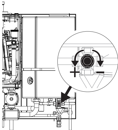
instellen thermostatisch mengventiel
