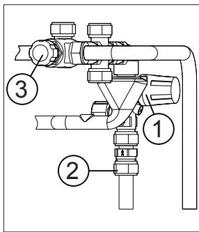
thermostatisch mengventiel, inlaatcombinatie en doseerventiel figuur 6.8.a
