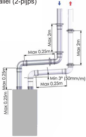
Beugelafstanden bij parallel aangesloten rookgasafvoer en luchttoevoer
