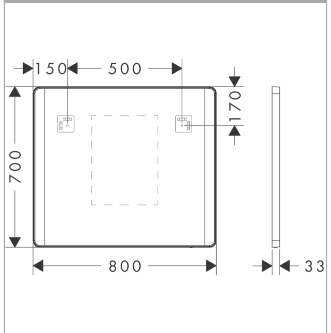
Maattekening
