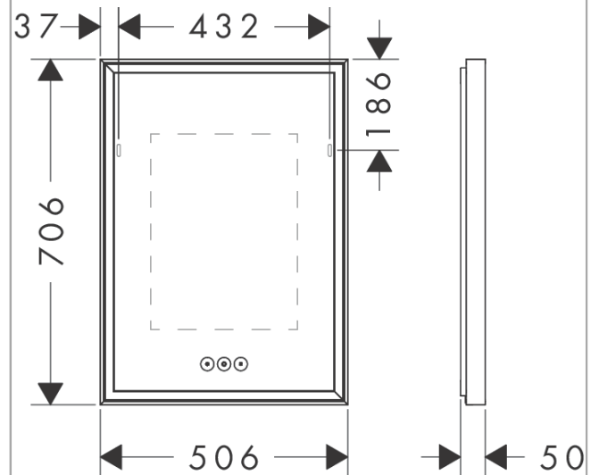
Maattekening
