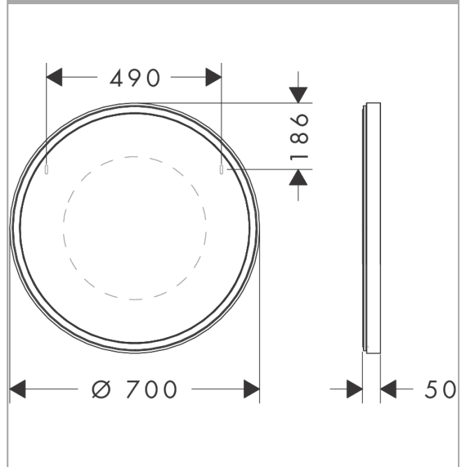
Maattekening
