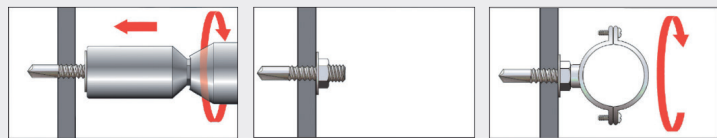
Metaalplaat
