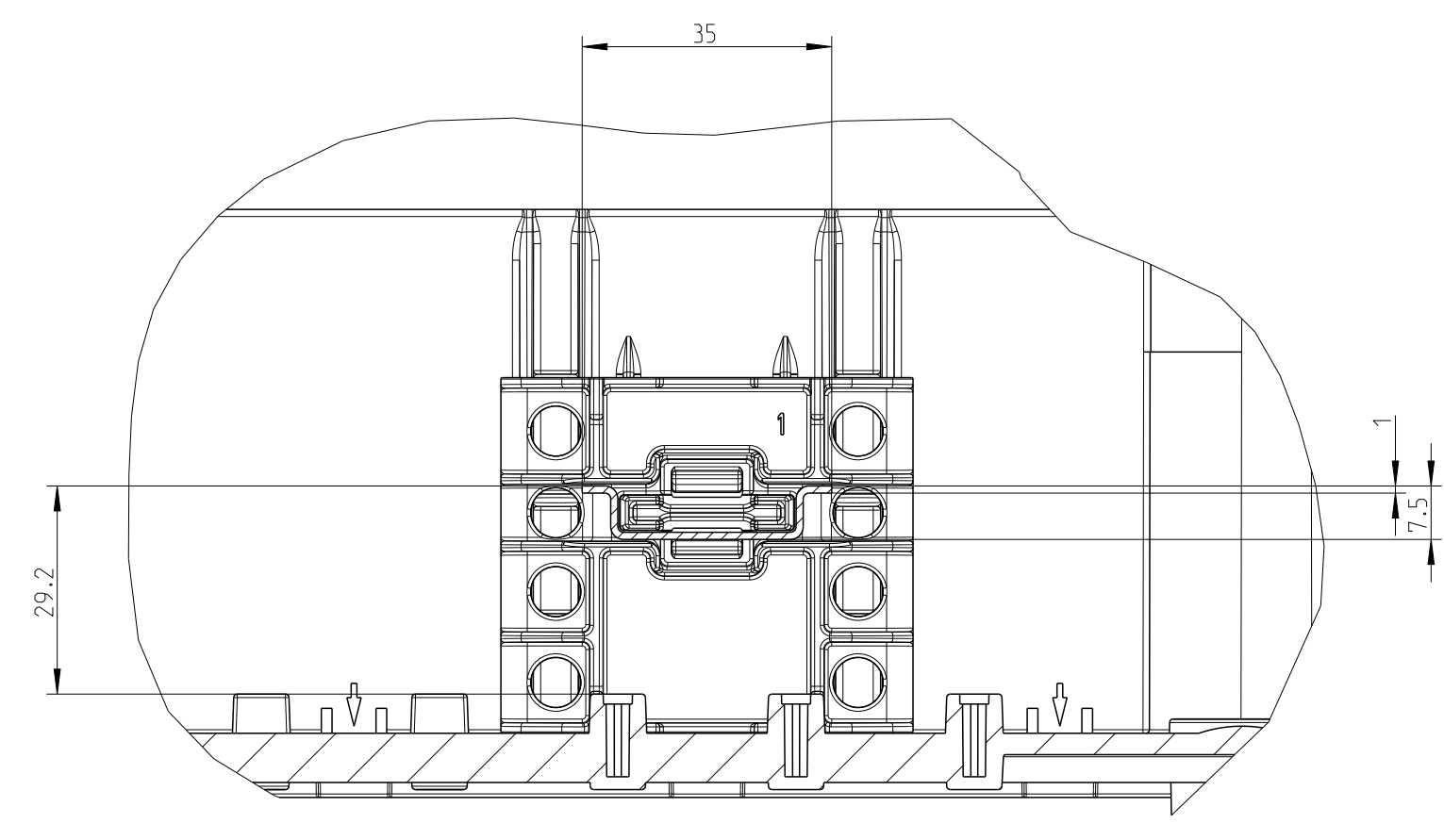
A-A Detail um 90° gedreht detail turned 90°
