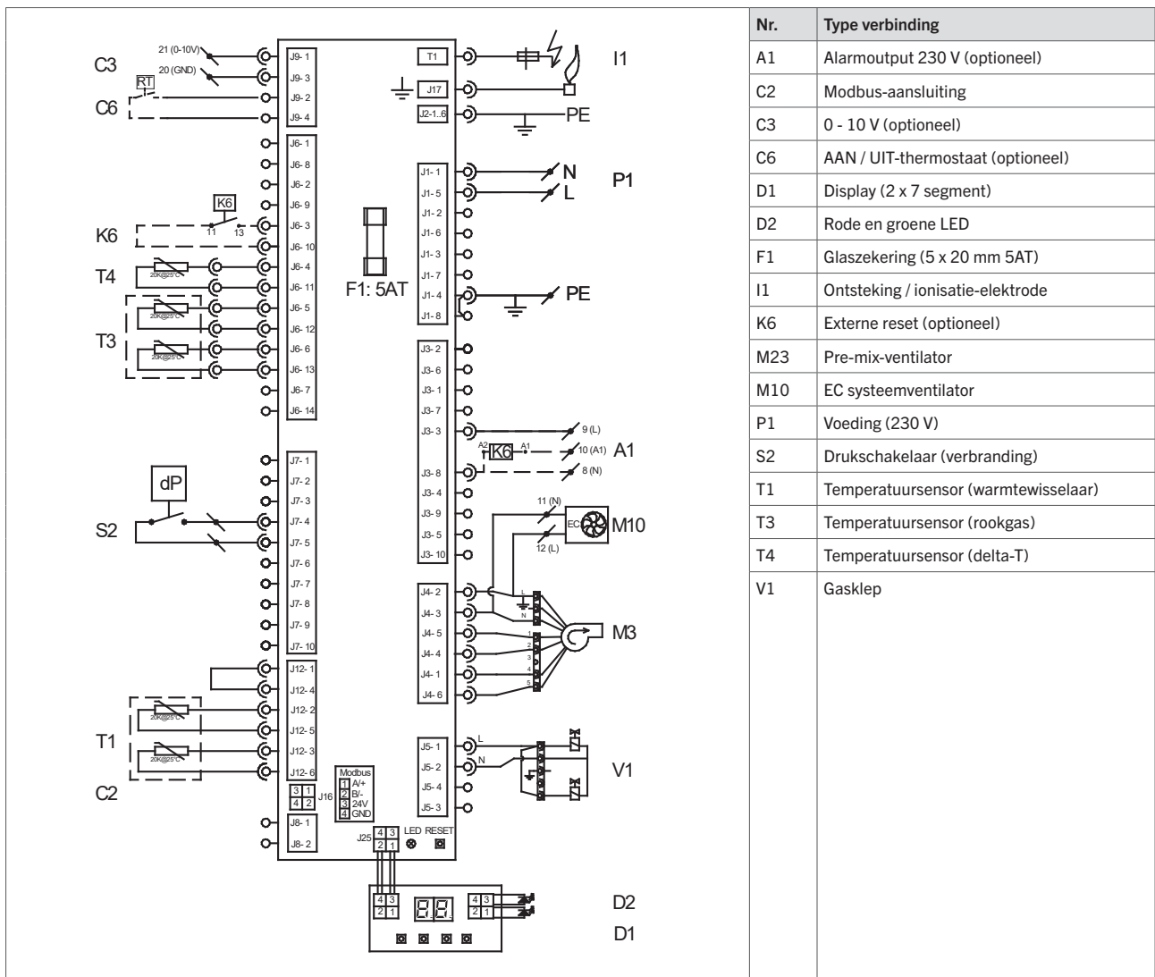
Figuur 25 - Elektrisch schema QSG
