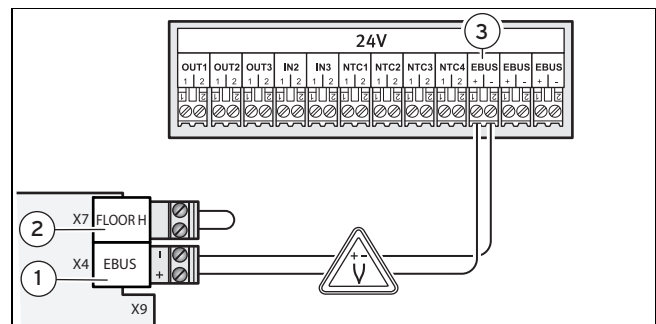
1 eBUS-aansluiting in de warmtepomp (op polariteit letten) 3 eBUS-aansluiting in de warmtepompbesturingsmodule 2 Aansluiting maximaalthermostaat (vloerveiligheidsschakeling)
