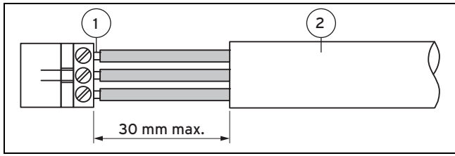
1 Aansluitdraden 2 Isolatie
