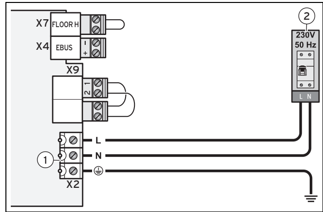
1 Netaansluitklemmen in het product 2 Ontkoppelinrichting
