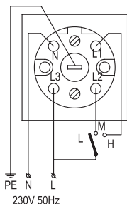
Perilex aansluiting
