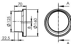
Sectie A-A
