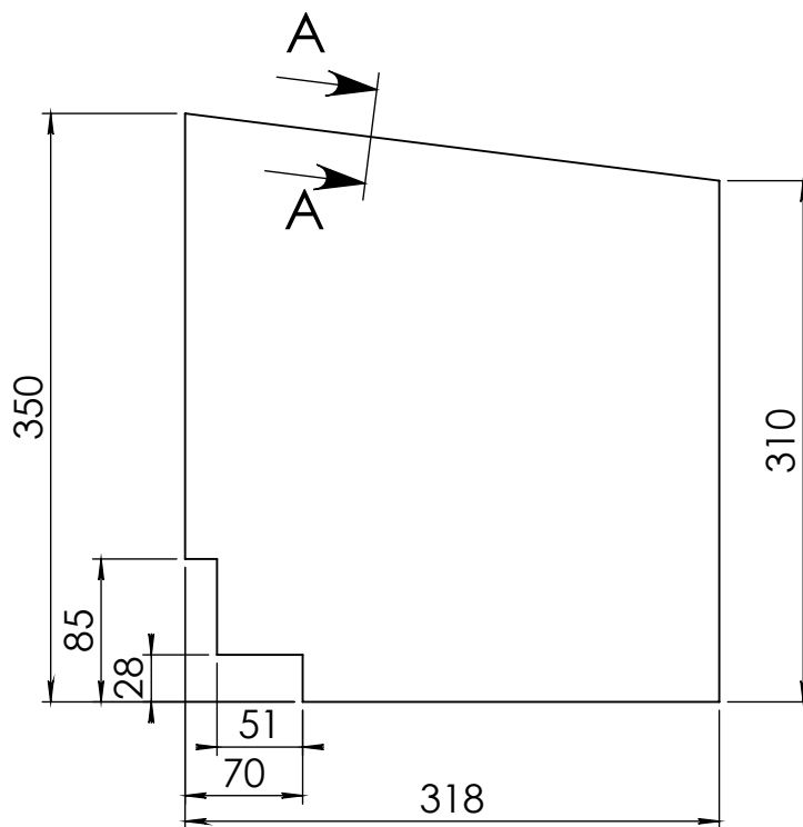
View A-A
