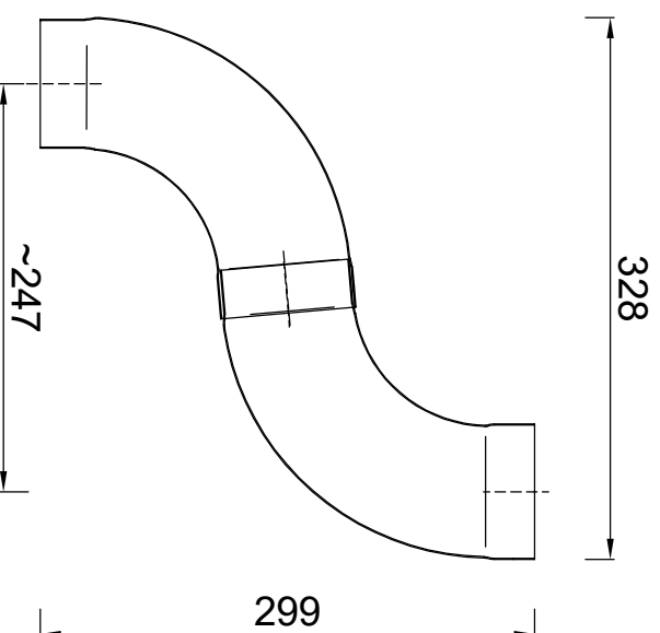
Doorsnede sprong
