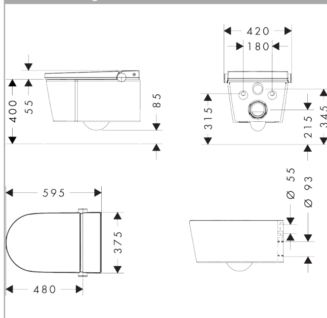
Maattekening
