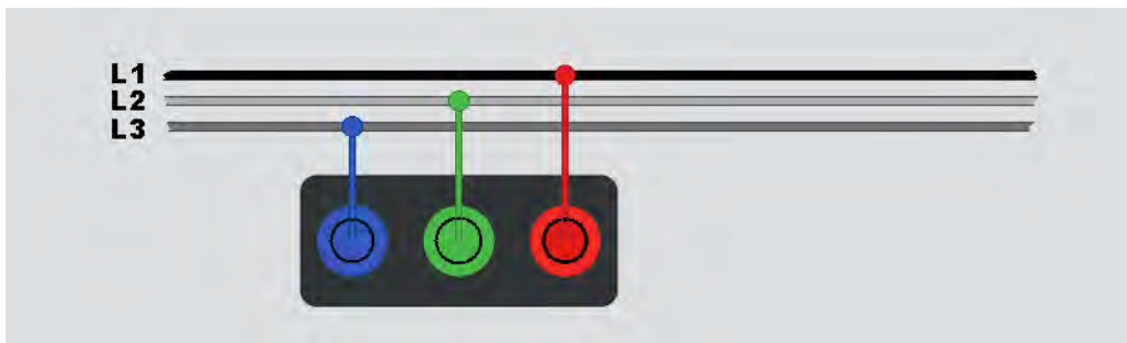
Afbeelding 19. Aansluiting voor faserotatietest
