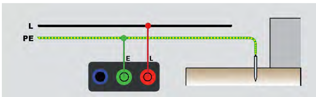
Afbeelding 25. 2-draads aansluiting voor lustest van aardingsweerstand (modus met uitschakeling, hoge stroomsterkte)
