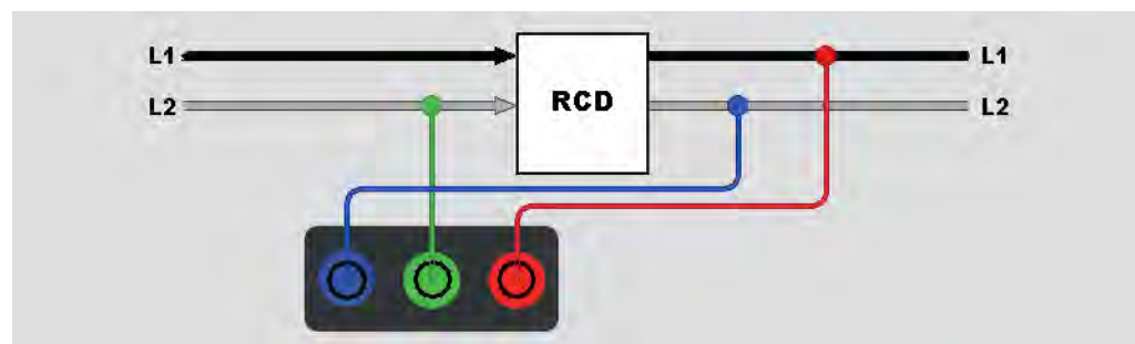
Afbeelding 17. Aansluiting voor het testen van ALS type B of ALS type A-EV in geïsoleerde geaarde elektrische systemen
