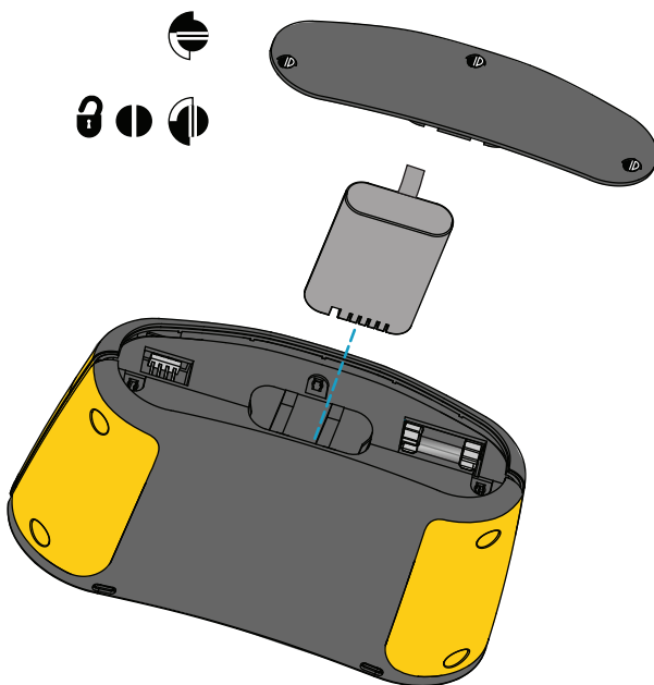
Afbeelding 28. Batterijen vervangen
