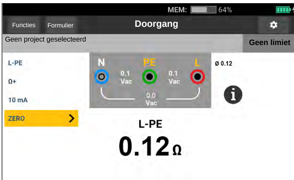
Afbeelding 6. Nulstellingsdisplay
