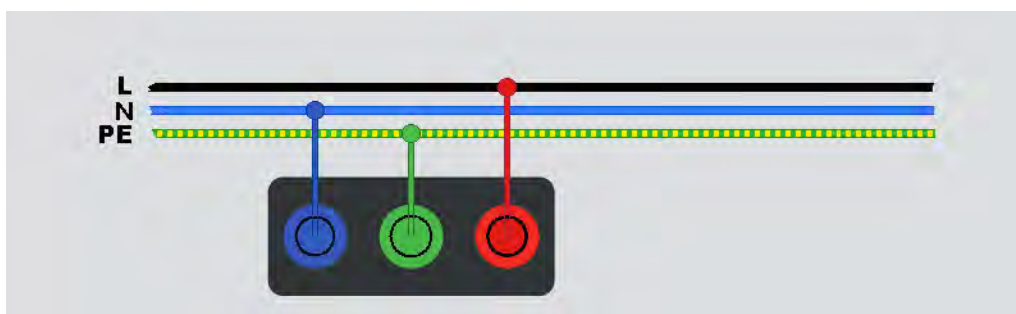
Afbeelding 24. 3-draads aansluiting voor lustest van aardingsweerstand (modus zonder uitschakeling)
