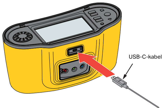
Afbeelding 27. USB-C-kabel aansluiten
