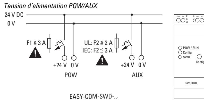
Fig. 345: EASY-COM-SWD-...Raccordement de la tension d'alimentation
