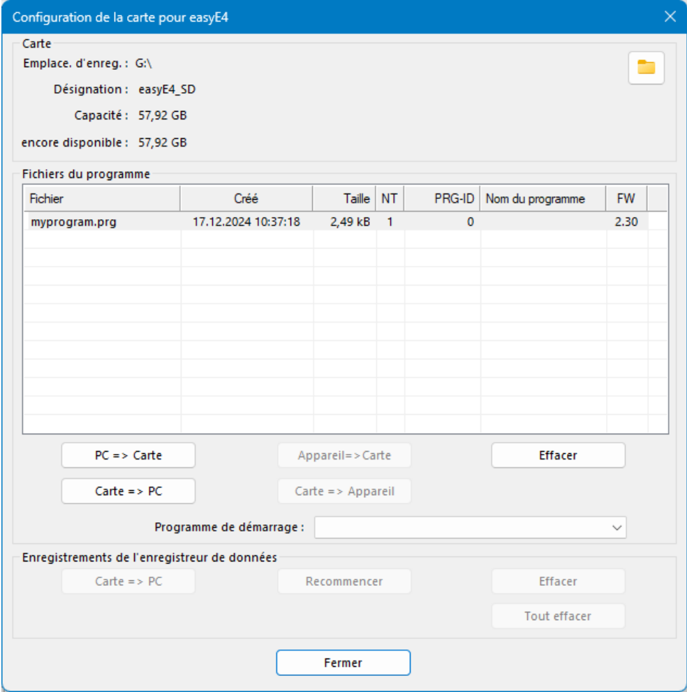
Fig. 70: Boîte de dialogue hors ligne carte mémoire
