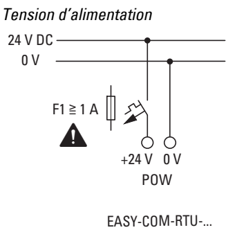
Fig. 351: EASY-COM-RTU-...Raccordement de la tension d'alimentation
