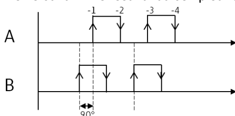
Fig. 176: Module fonctionnel CI à comptage dans l'ordre décroissant ; QV=QV-4
