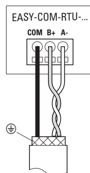
Fig. 350: Raccordement des sorties EASY-COM-RTU-...
