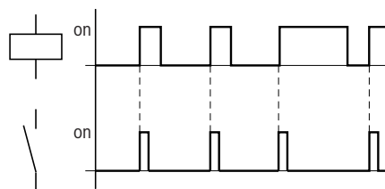
Fig. 102: Diagramme fonctionnel d'une "impulsion sur un cycle" en cas de front montant
