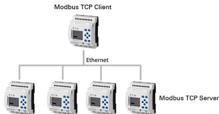
Fig. 382: Exemple : easyE4 comme client Modbus TCP
