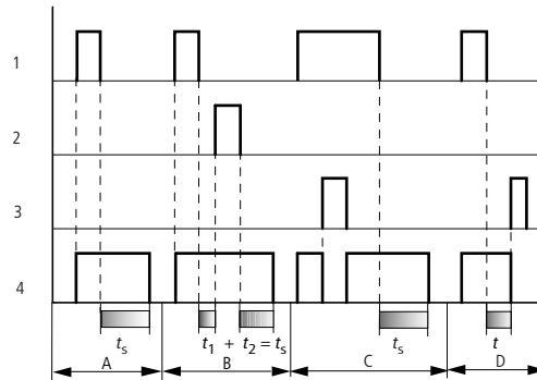
Fig. 147: Diagramme fonctionnel Relais temporisé avec retard à la chute (avec/sans commutation, avec/sans réactivation)
