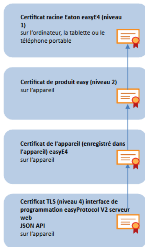
Fig. 316: Chaîne de certificats easyE4
