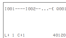
Fig. 84: Schéma avec entrées I 01, I 02 et sortie Q 1
