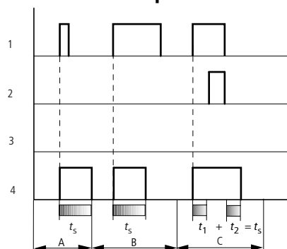
Fig. 150: Diagramme fonctionnel n° 1 d'un relais temporisé avec mise en forme d'une impulsion
