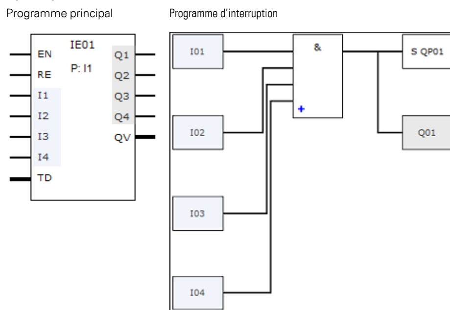
Fig. 266: Transmission des états des entrées et sorties entre le programme principal et le programme d'interruption
