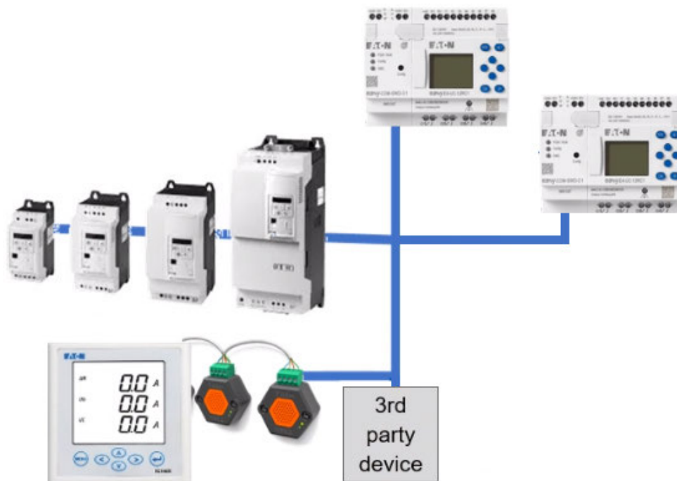
Fig. 348: Synoptique : easyE4 comme maître Modbus RTU communique avec DE1, DC1, DG1, DA1, easyE4 comme esclave Modbus RTU et autres appareils
