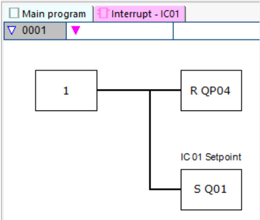
Fig. 259: Programme d'interruption easySoft 8 compteur d'impulsions avec direction externe
