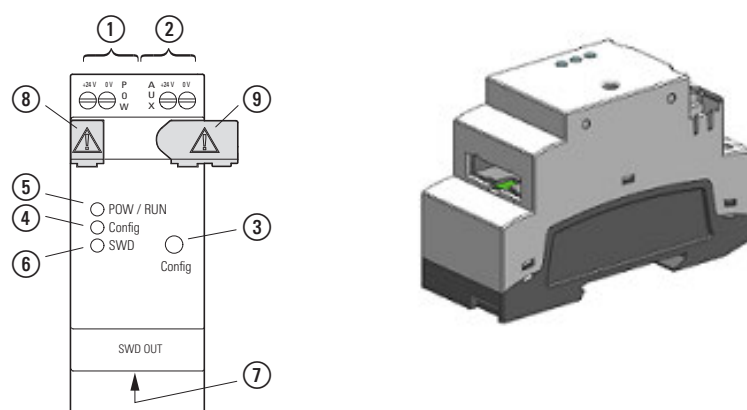
Fig. 344: Version de l'appareil avec 2 PE
