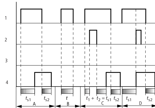
Fig. 149: Diagramme fonctionnel d'un relais temporisé retardé à l'appel et à la chute
