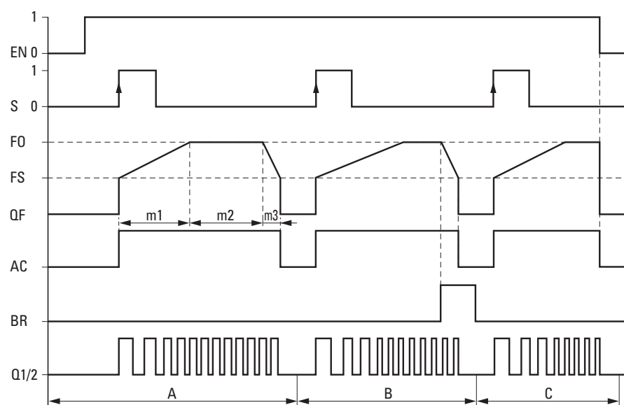
Fig. 199: Diagramme fonctionnel Émission d'impulsions PO avec nombre d'impulsions I1 prédéfini - phases possibles du mode de fonctionnement normal
