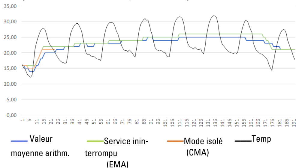
Fig. 182: Exemple de courbe caractéristique horaire, sur 7 jours
