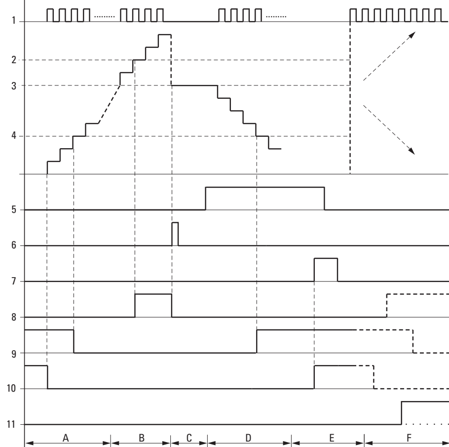
Fig. 174: Diagramme fonctionnel compteur rapide
