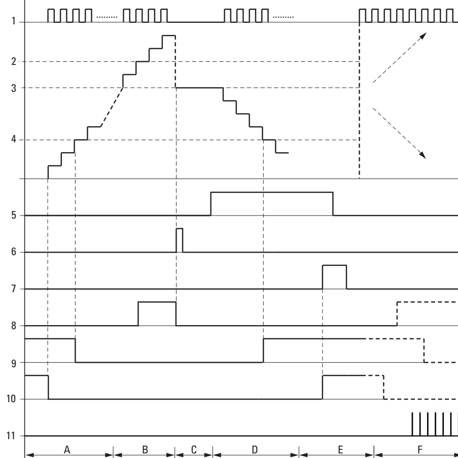
Fig. 177: Diagramme fonctionnel compteur incrémental rapide
