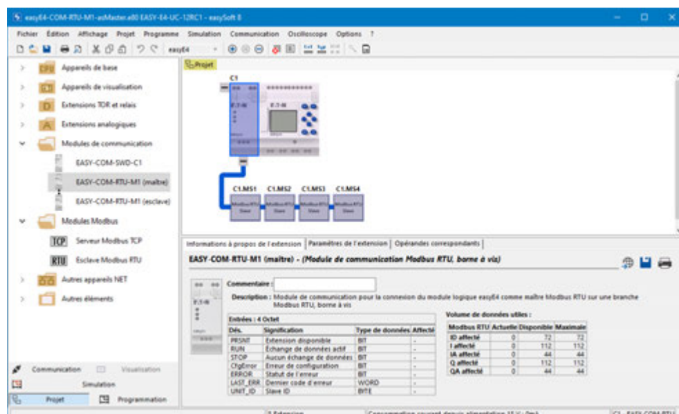
Fig. 352: Zone de travail avec appareil de base et module de communication EASY-COM-RTU-M1 maître
