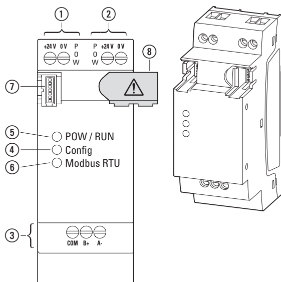
Fig. 349: Synoptique des appareils easy
