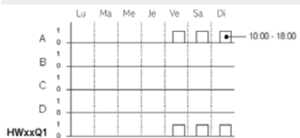
Fig. 126: Diagramme fonctionnel
