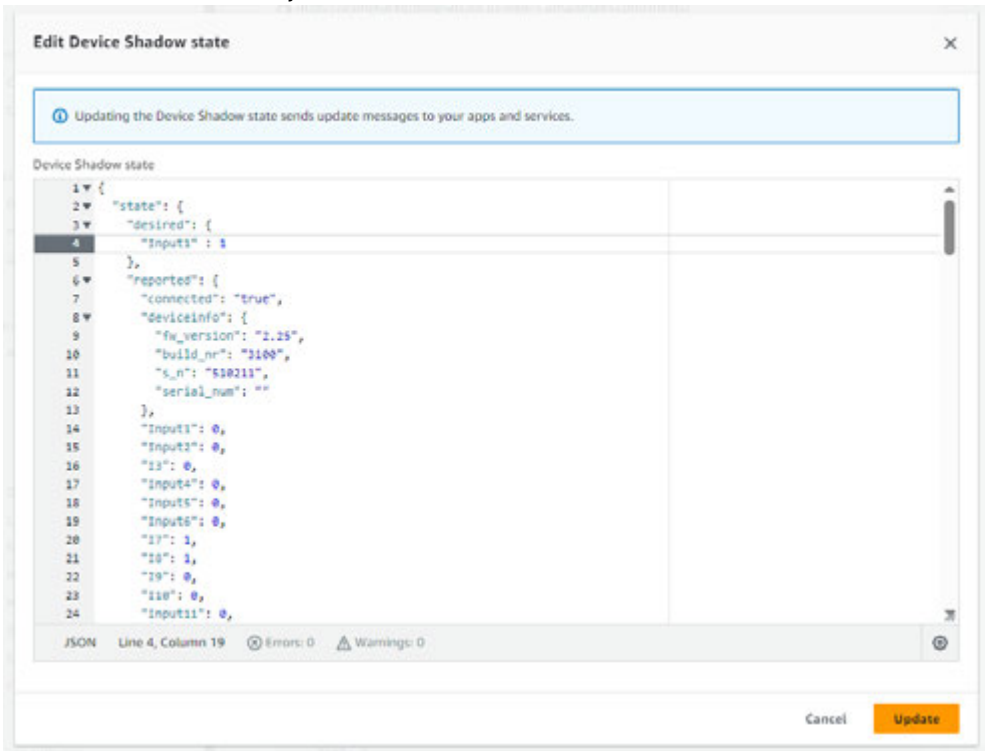
Fig. 359: Exemple : onglet AWS Device Classic Shadow, éditeur
