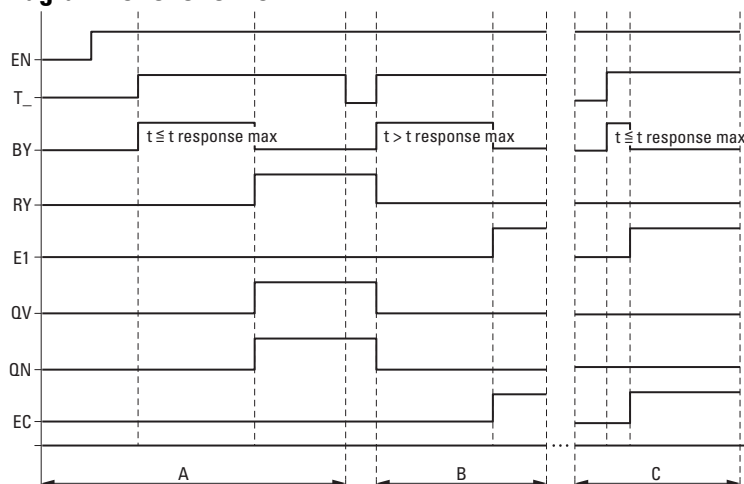
Fig. 252: Diagramme fonctionnel d'un compteur de fréquence
