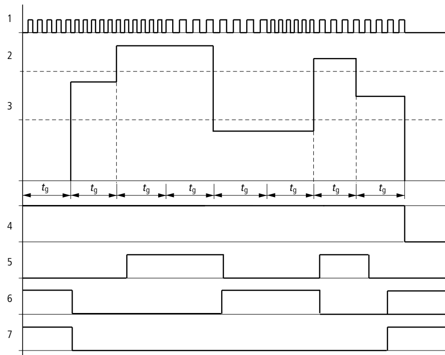
Fig. 173: Diagramme fonctionnel d'un compteur de fréquence
