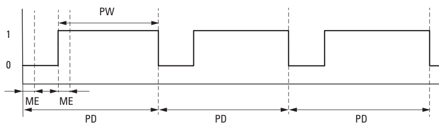
Fig. 190: Impulsions PW sur la sortie du module avec SV = 3218, ME = 93 ms, PD = 1000 ms
