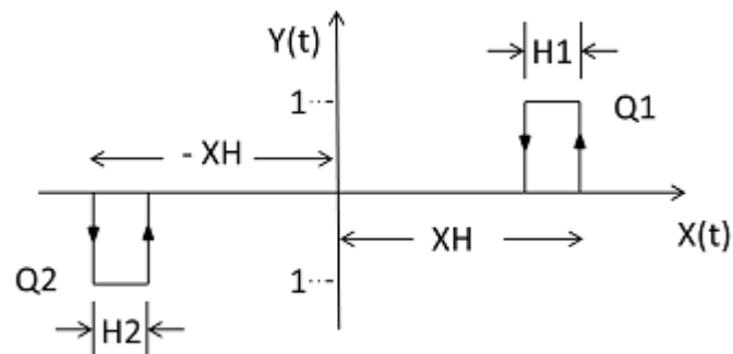
Fig. 204: Diagramme des temps du régulateur à trois points
