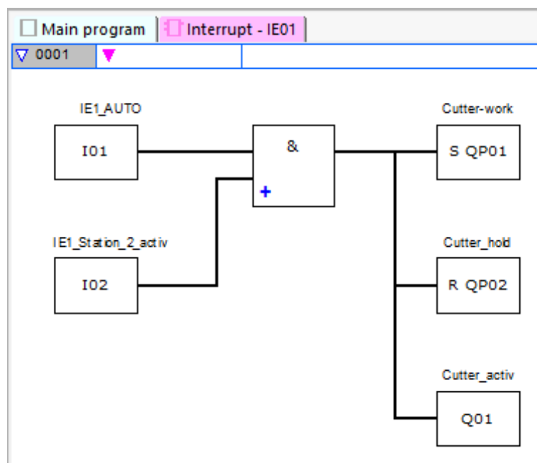
Fig. 268: Programme d'interruption easySoft 8 à commande par fronts
