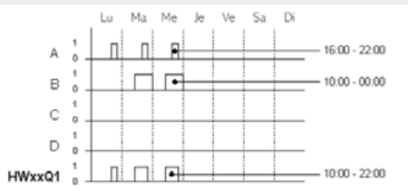
Fig. 132: Diagramme fonctionnel
