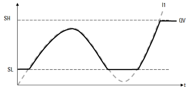
Fig. 206: Figure : Limitation des valeurs d'entrée aux limites prédéterminées
