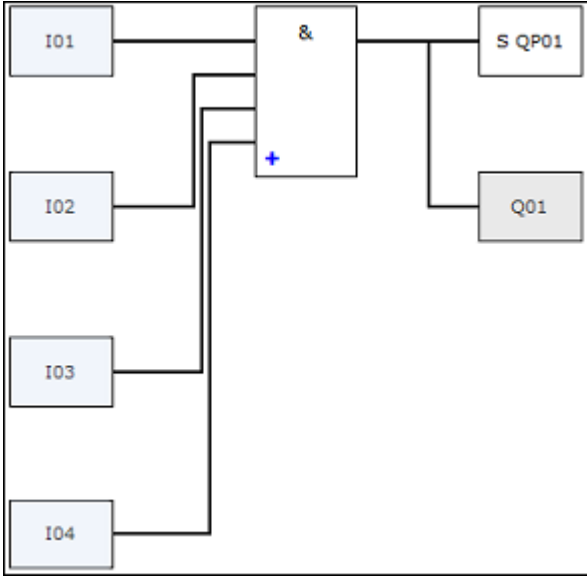
Fig. 269: Transmission des états des entrées et sorties entre le programme principal et le programme d'interruption
