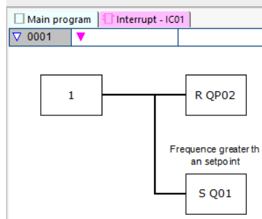
Fig. 265: Programme d'interruption easySoft 8 mesure de fréquence
