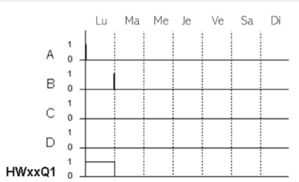
Fig. 134: Diagramme fonctionnel
