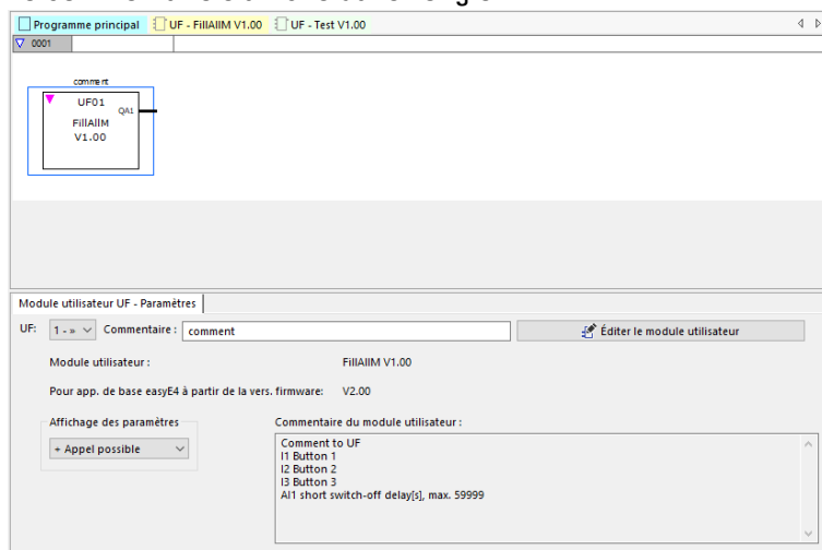
Fig. 277: Commentaire du module utilisateur affiché dans l'onglet
