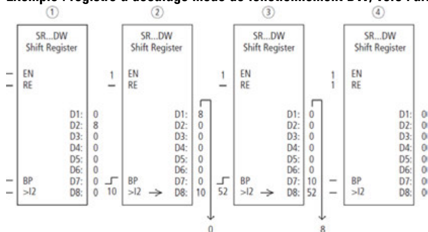
Fig. 220: Registre à décalage SR.. : opération de décalage vers l'arrière en mode DW
