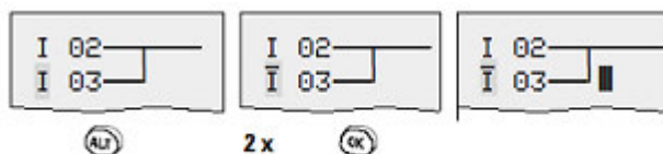
Fig. 106: Passage du contact à fermeture I 03 en contact à ouverture
