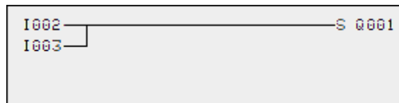
Fig. 116: Raccordement en parallèle
