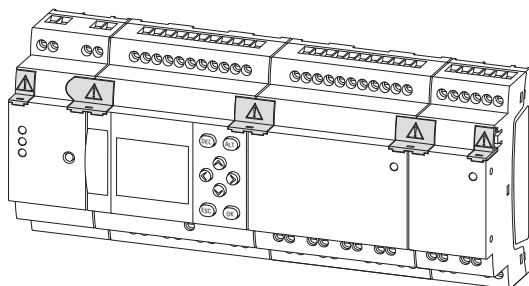
Fig. 343: Exemple module logique easyE4 avec extensions E/S et module de communication easy EASY-COM-SWD-...
