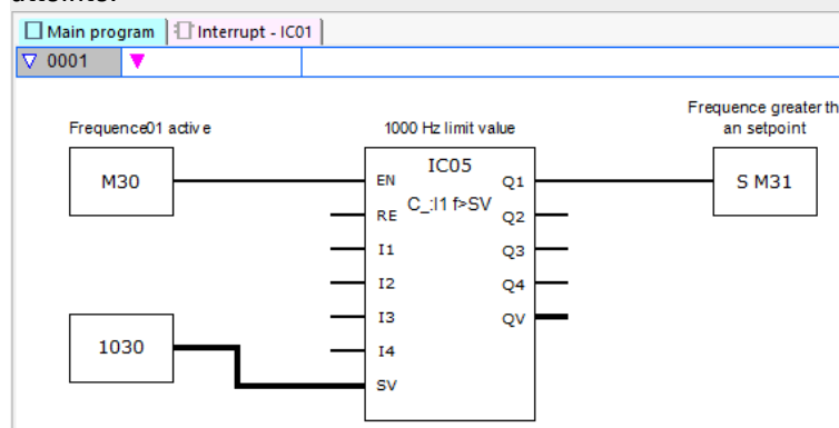
Fig. 264: Programme principal easySoft 8 mesure de fréquence
