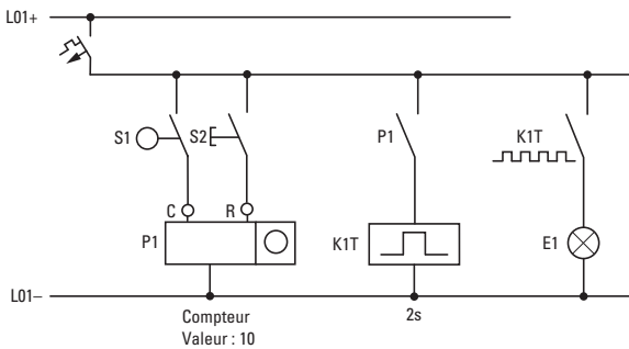
Fig. 290: Câblage fixe avec relais
