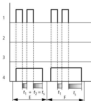
Fig. 148: Diagramme fonctionnel Relais temporisé avec retard à la chute (avec/sans commutation, avec/sans réactivation)
