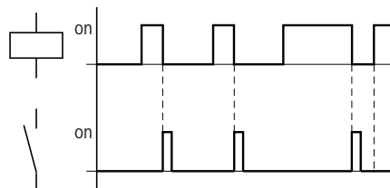
Fig. 103: Diagramme fonctionnel d'une "impulsion sur un cycle" en cas de front descendant
