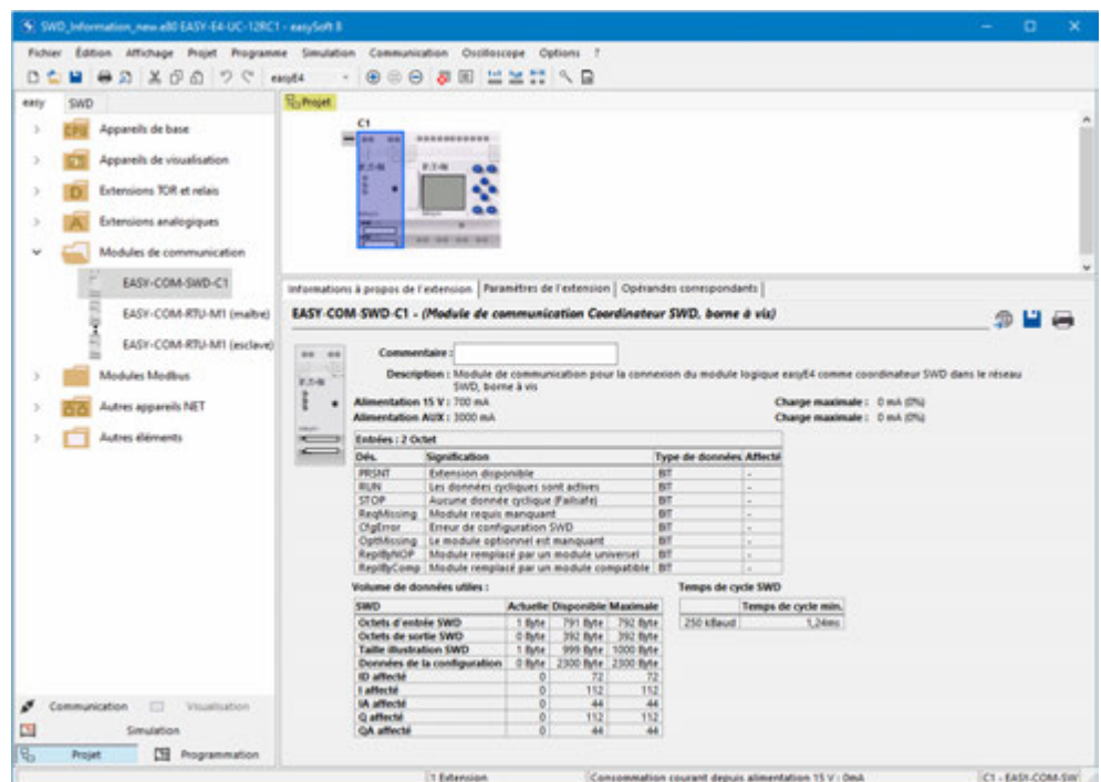
Fig. 347: Zone de travail avec appareil de base et module de communication, catalogue d'appareils étendu avec l'onglet "SWD"
