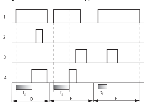
Fig. 146: Diagramme fonctionnel d'un relais temporisé retardé à l'appel (avec/sans commutation aléatoire)
