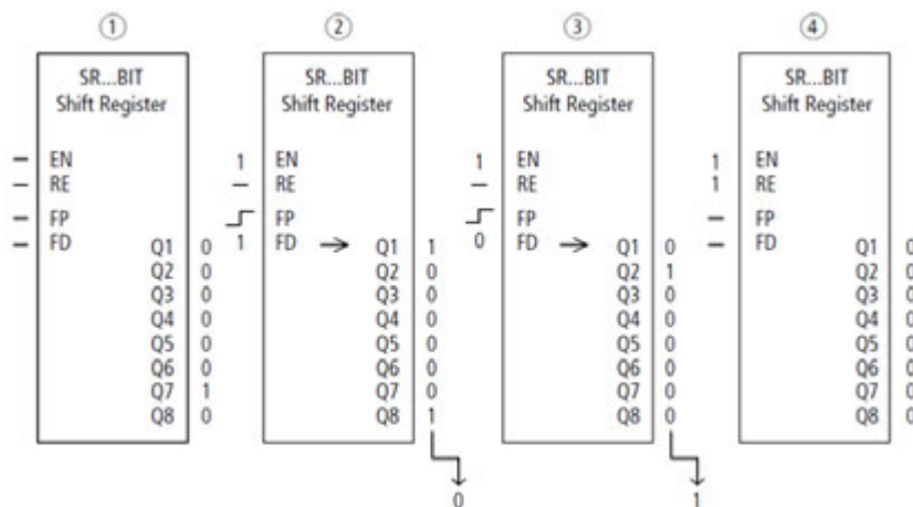
Fig. 219: Registre à décalage SR.. : opération de décalage vers l'avant en mode BIT
