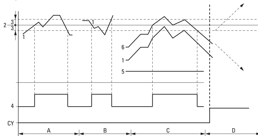
Fig. 178: Diagramme fonctionnel comparateur de valeurs analogiques
