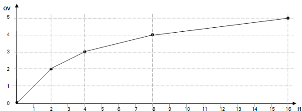
Fig. 188: Exemple de courbe caractéristique pour module fonctionnel PM
