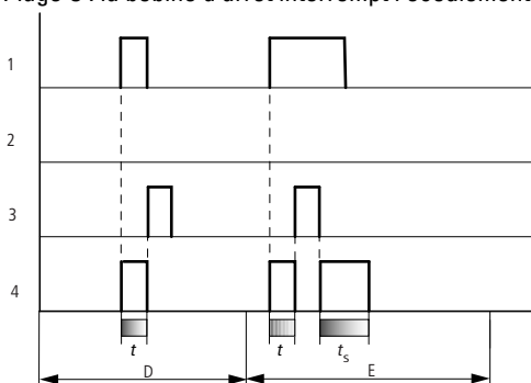
Fig. 151: Diagramme fonctionnel n° 2 d'un relais temporisé avec mise en forme d'une impulsion
