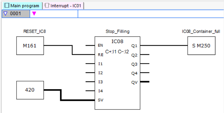
Fig. 260: Programme principal easySoft 8 deux entrées de comptage
