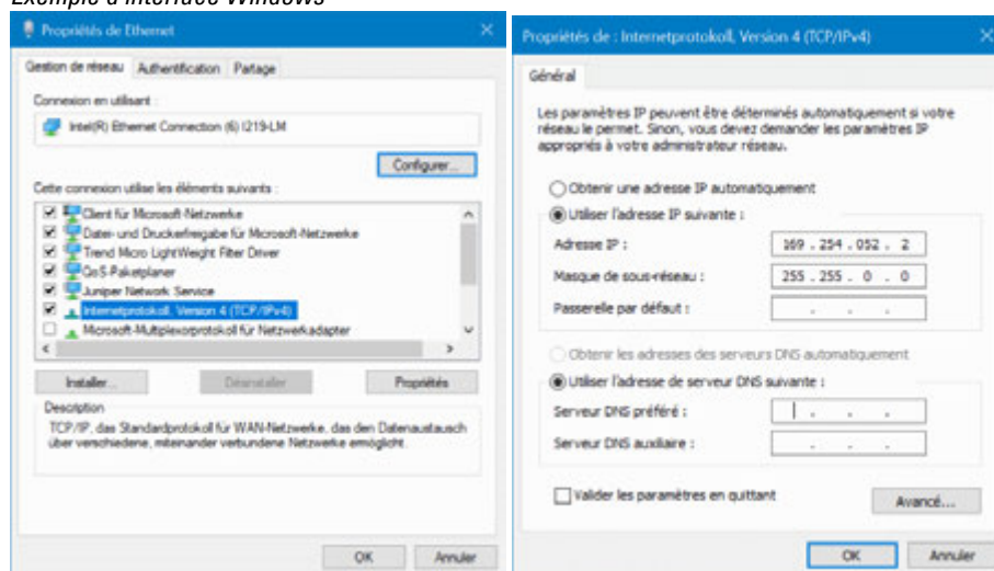
Fig. 95: Connexion Ethernet sur l'ordinateur
