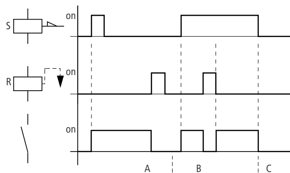
Fig. 99: Diagramme fonctionnel des fonctions "Bobine d'accrochage" et "Bobine de décrochage"
