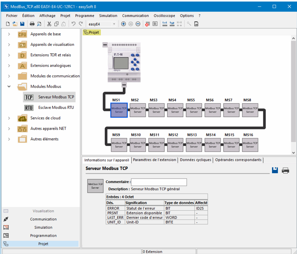
Fig. 384: Zone de travail avec appareil de base et modules Serveur Modbus TCP
