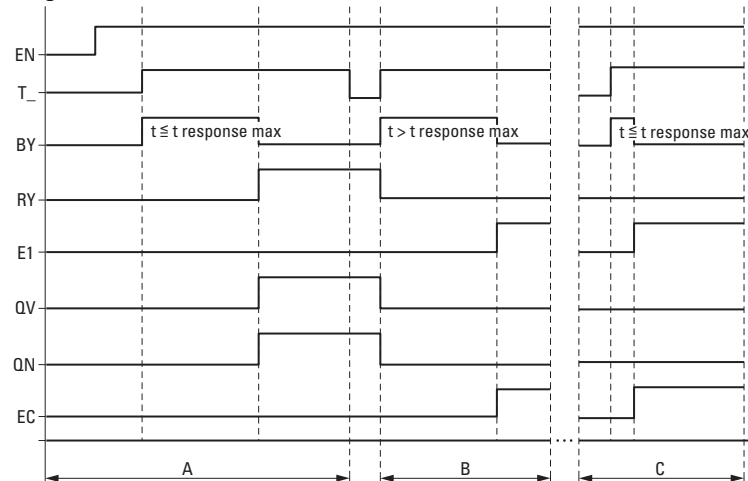
Fig. 242: Diagramme fonctionnel d'un compteur de fréquence
