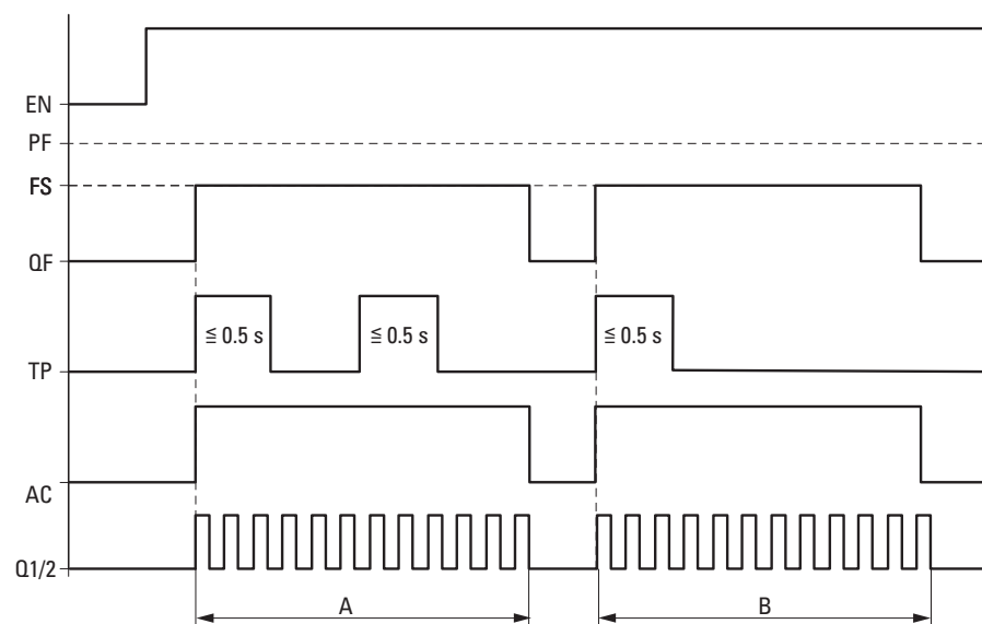
Fig. 200: Diagramme fonctionnel mode pianotage avec nombre de pas P1 prédéfini
