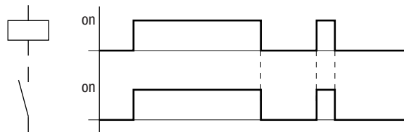
Fig. 97: Diagramme fonctionnel d'une bobine avec fonction contacteur
