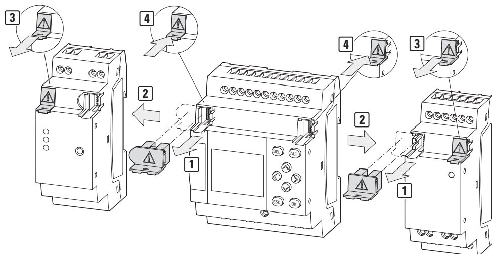
Fig. 15: Retirer les connecteurs de liaison voisins
