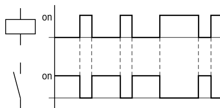
Fig. 101: Diagramme fonctionnel de la "fonction contacteur inversée"
