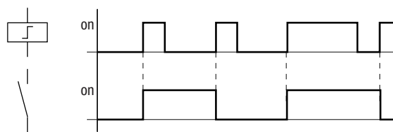
Fig. 98: Diagramme fonctionnel d'un "relais avec fonction télérupteur"
