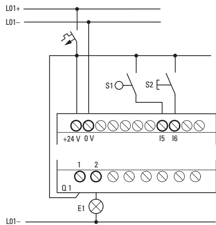
Fig. 291: Câblage p. ex. avec EASY-E4-UC-...
