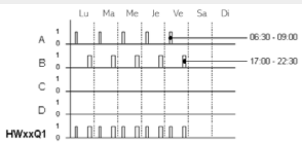
Fig. 128: Diagramme fonctionnel
