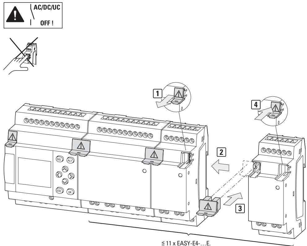
Fig. 10: Montage de l'appareil de base avec extensions
