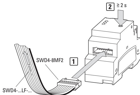
Fig. 346: EASY-COM-SWD-... Raccordement
