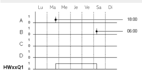
Fig. 130: Diagramme fonctionnel
