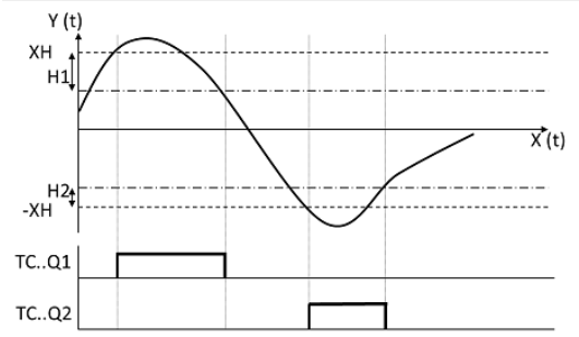
Fig. 205: Diagramme fonctionnel du régulateur à trois points
