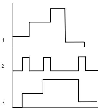
Fig. 214: Diagramme fonctionnel module de données
