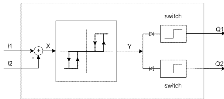
Fig. 203: Schéma de principe du régulateur à trois points
