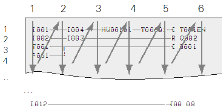
Fig. 303: Comment EDP évalue le schéma et les modules fonctionnels easy
