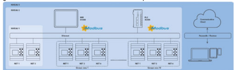
Fig. 318: Synoptique NET
