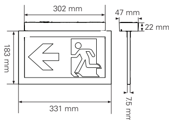
Seilabhängungs-Set
