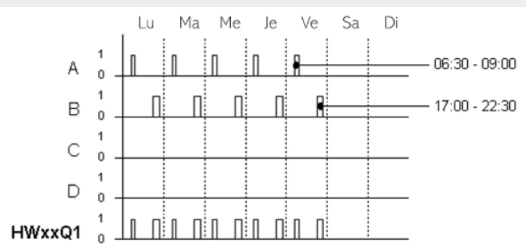
Fig. 127: Diagramme fonctionnel
