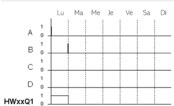
Fig. 133: Diagramme fonctionnel
