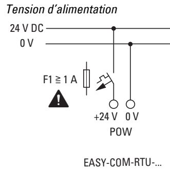
Fig. 348: Raccordement de la tension d'alimentation EASY-COM-RTU-...
