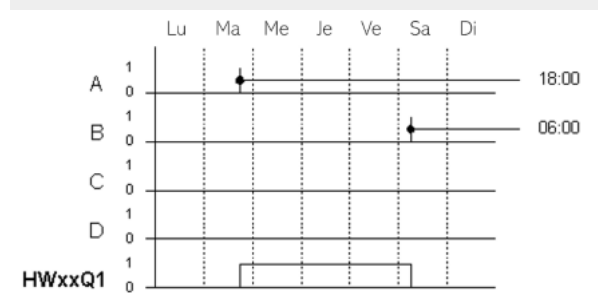
Fig. 129: Diagramme fonctionnel
