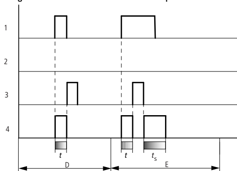
Fig. 150: Diagramme fonctionnel n° 2 d'un relais temporisé avec mise en forme d'une impulsion
