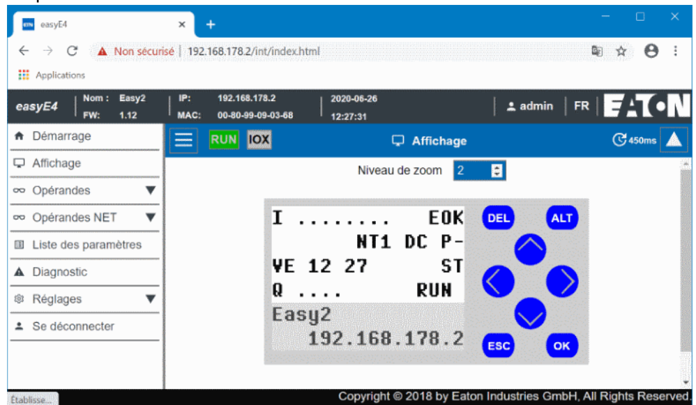
Fig. 324: Afficheur de l'appareil
