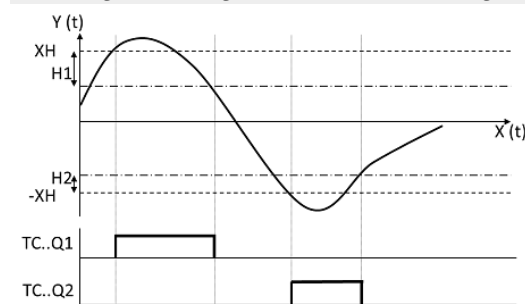
Fig. 204: Diagramme fonctionnel du régulateur à trois points
