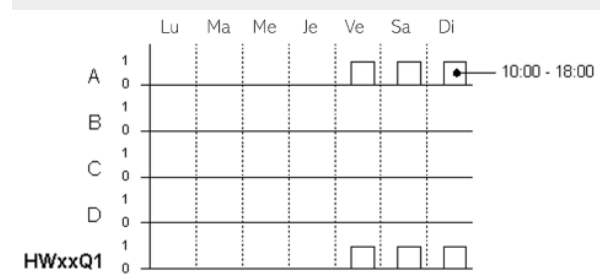
Fig. 125: Diagramme fonctionnel
